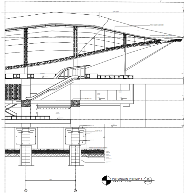
Gambar 6. 11 Potongan Prinsip 1 (Sumber : Dokumen Pribadi)
