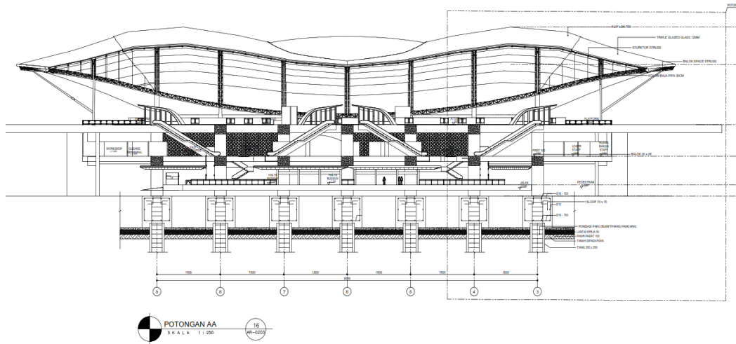
Gambar 6. 9 Potongan A (Sumber : Dokumen Pribadi)
