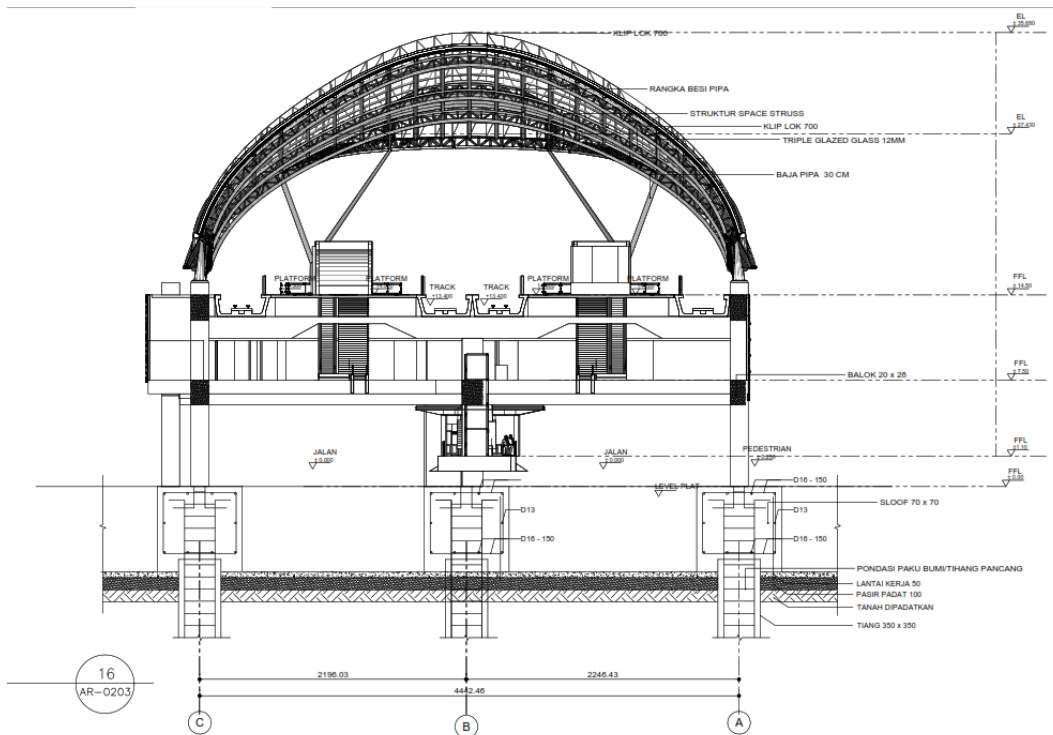
Gambar 6. 10 Potongan B (Sumber : Dokumen Pribadi)
