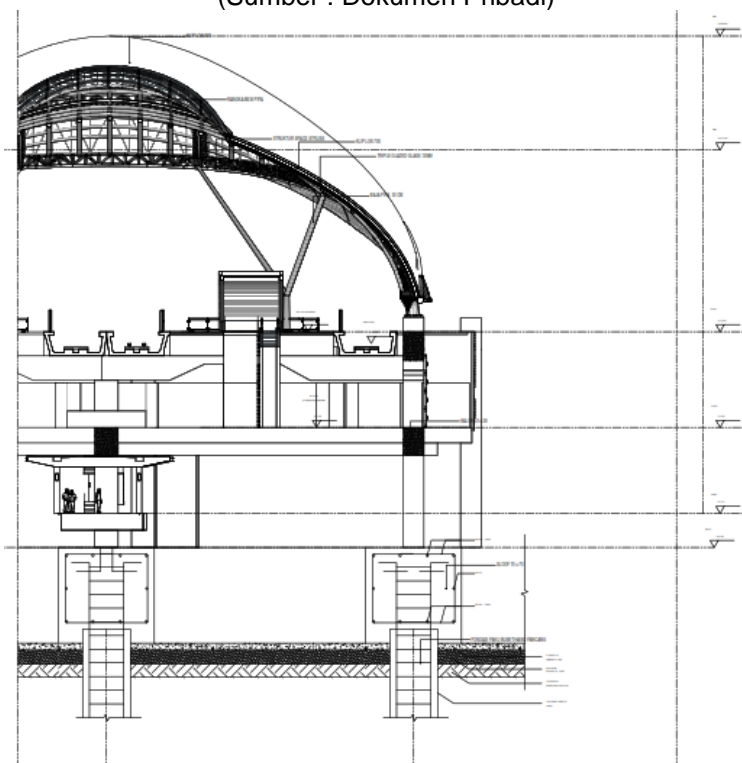
Gambar 6. 12 Poongan Prinsip 2 (Sumber : Dokumen Pribadi)
