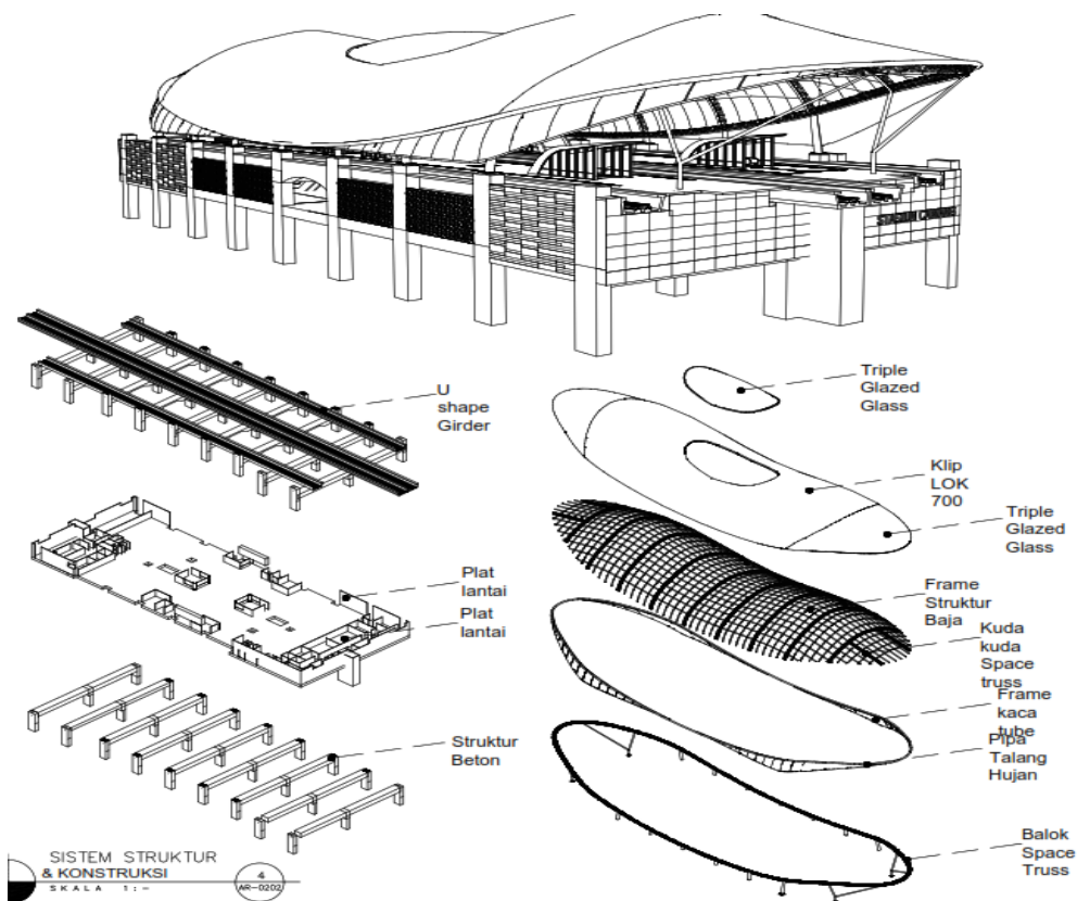
Gambar 6. 13 Sisitem Struktur (Sumber : Dokumen Pribadi)
