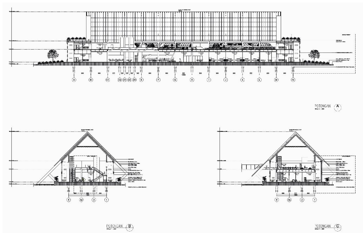
Gambar 6. 6 Potongan A-A, B-B dan C-C
