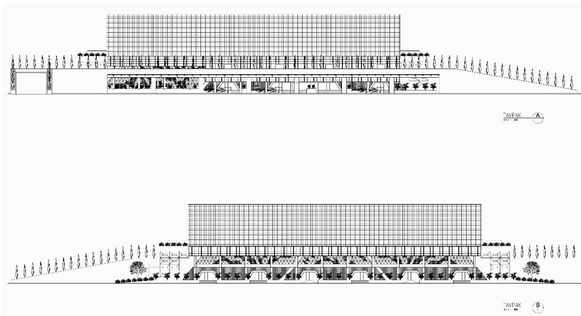
Gambar 6. 5 Tampak A dan B
