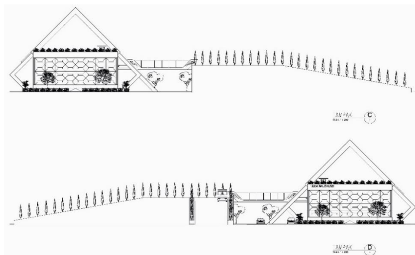
Gambar 6. 4 Tampak C dan D Sumber : Data pribadi
