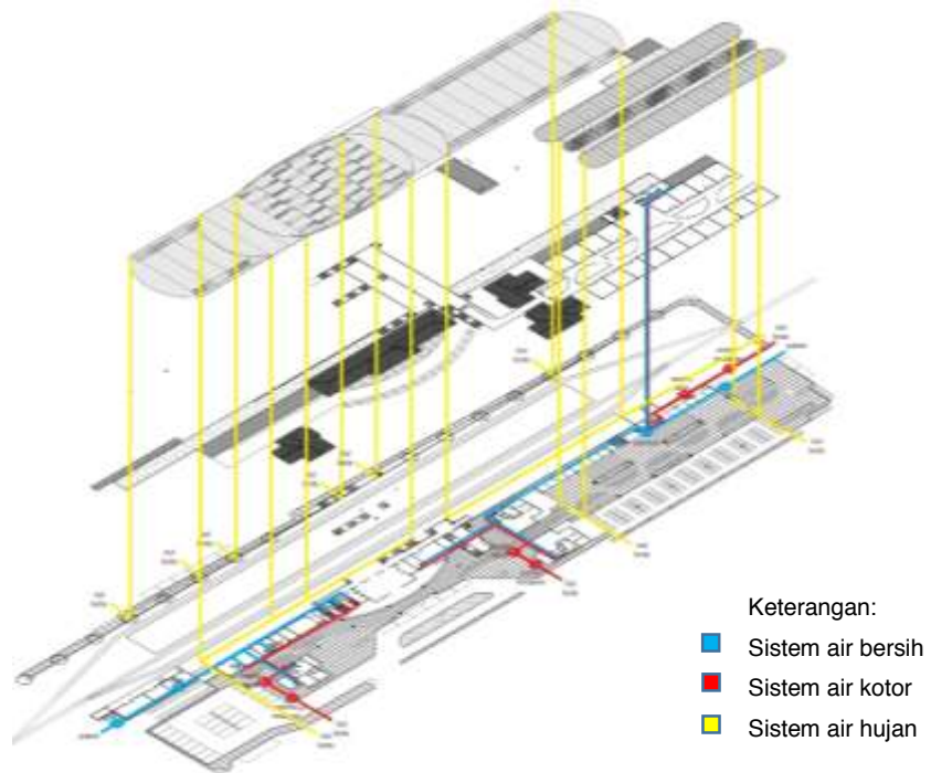
Gambar 6.14 Isometri sistem utilitas
