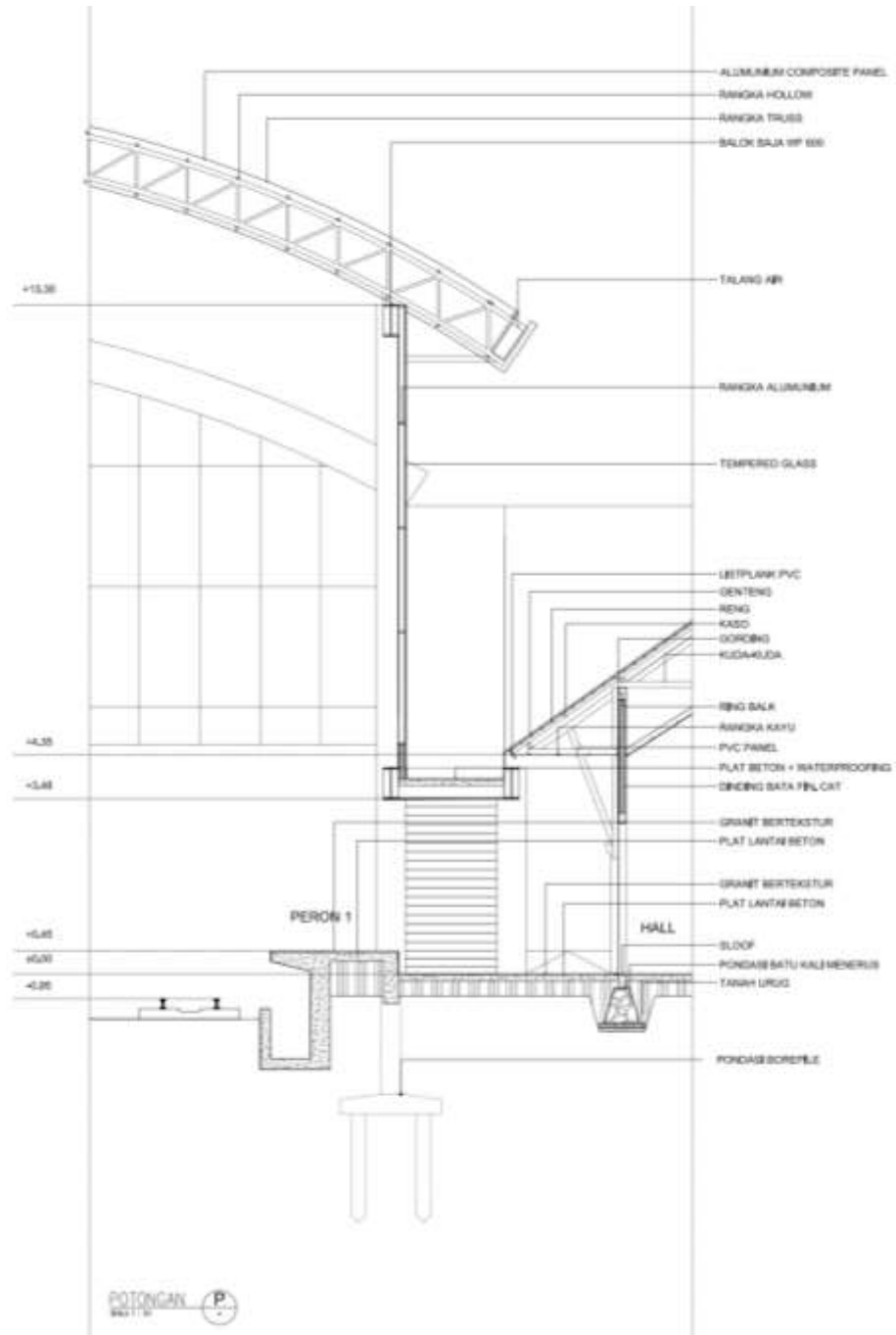
Gambar 6.12 Potongan Prinsip
