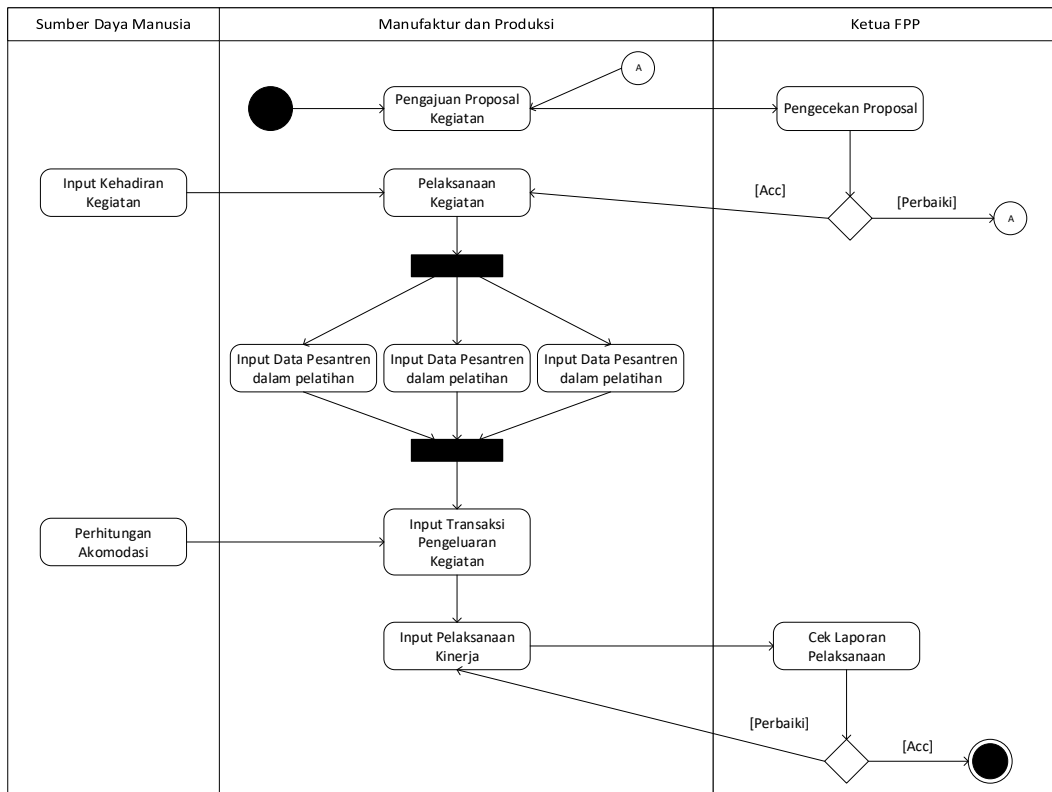
Gambar 4.11 Sub Activity Manufaktur dan Produksi
