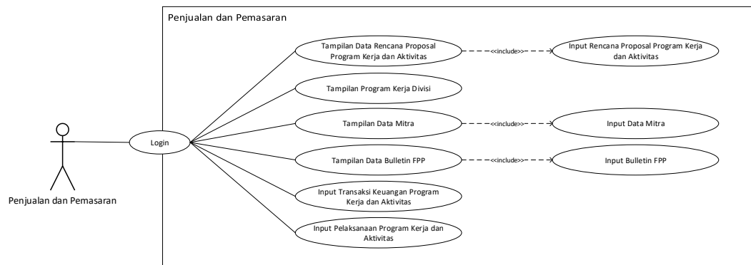
Gambar 4.8 Use Case Diagram Package Penjualan dan Pemasaran
