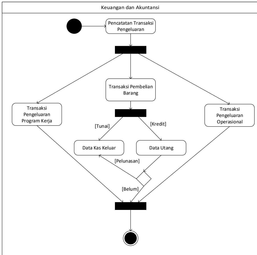
Gambar 4.13 Sub Activity Transaksi Pengeluaran
