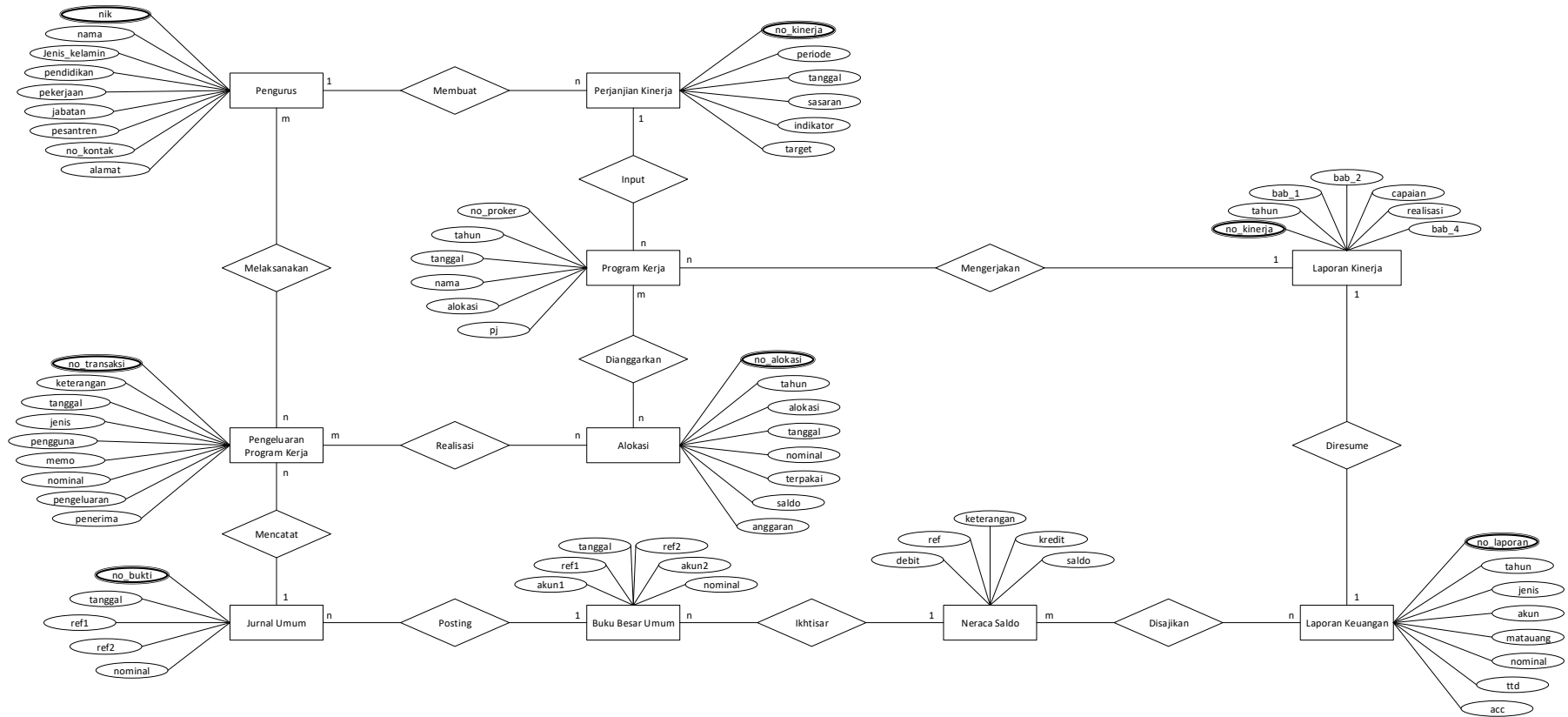
Gambar 4.15 Entity Relationship Diagram yang diusulkan
