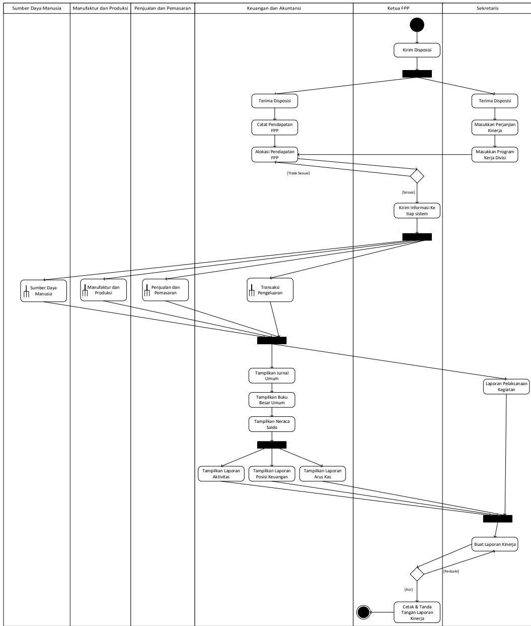
Gambar 4.9 Activity Diagram yang diusulkan
