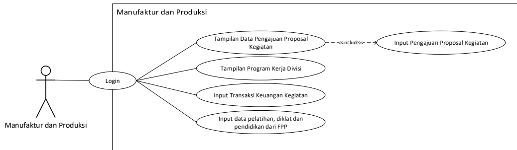
Gambar 4.7 Use Case Diagram Package Manufaktur dan Produksi
