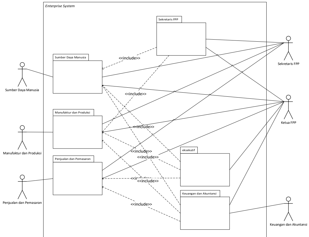
Gambar 4.2 Use Case Package Diagram yang diusulkan
