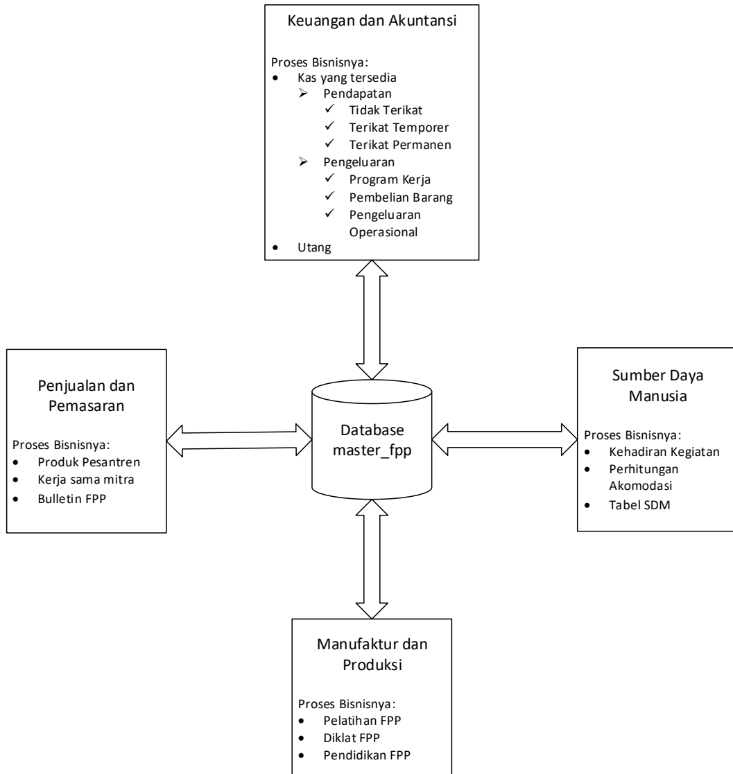
Gambar 4.1 Model Enterprise System FPP JABAR yang diusulkan
