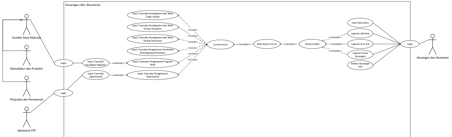
Gambar 4.5 Use Case Diagram Package Keuangan dan Akuntansi
