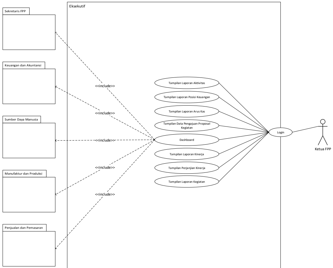
Gambar 4.3 Use Case Diagram Package Ketua FPP
