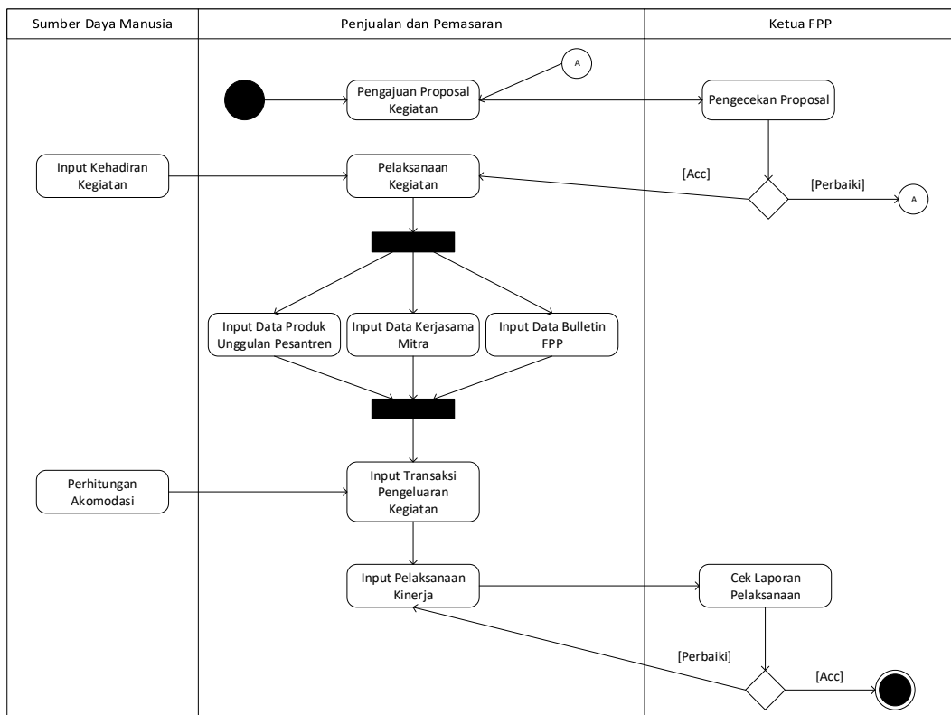
Gambar 4.12 Sub Activity Penjualan dan Pemasaran
