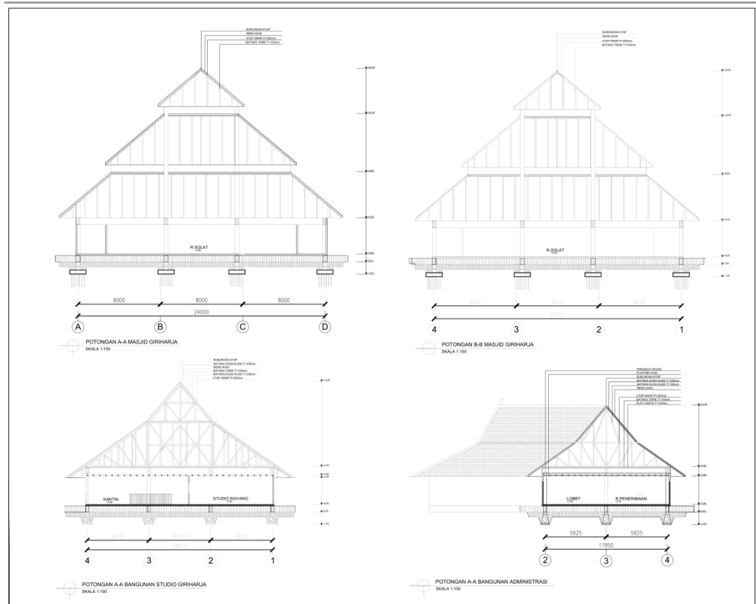
Gambar 6.10 Potongan Sumber : Pribadi
