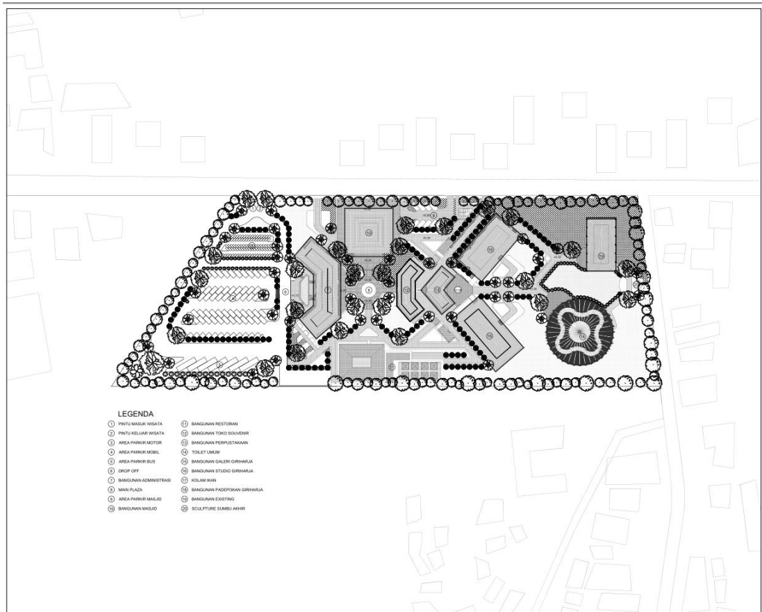
Gambar 6.3 Blok Plan Sumber : Pribadi
