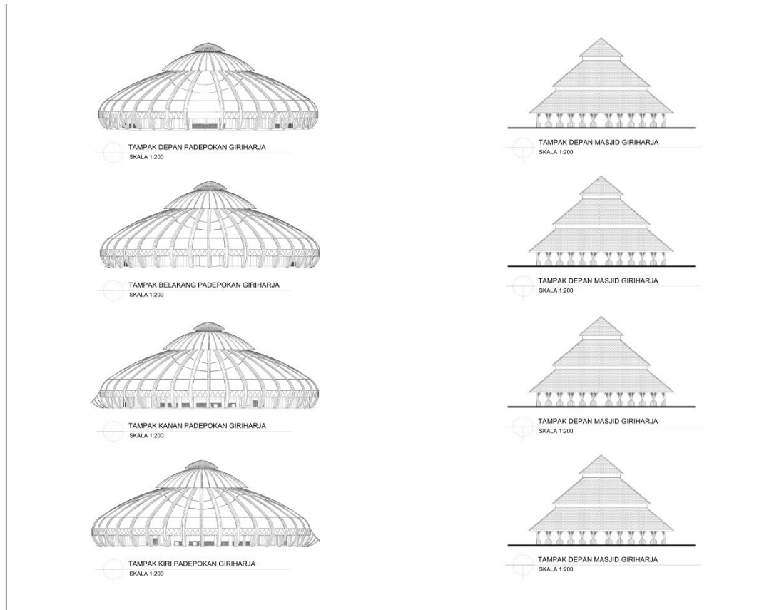
Gambar 6.6 Tampak Sumber : Pribadi
