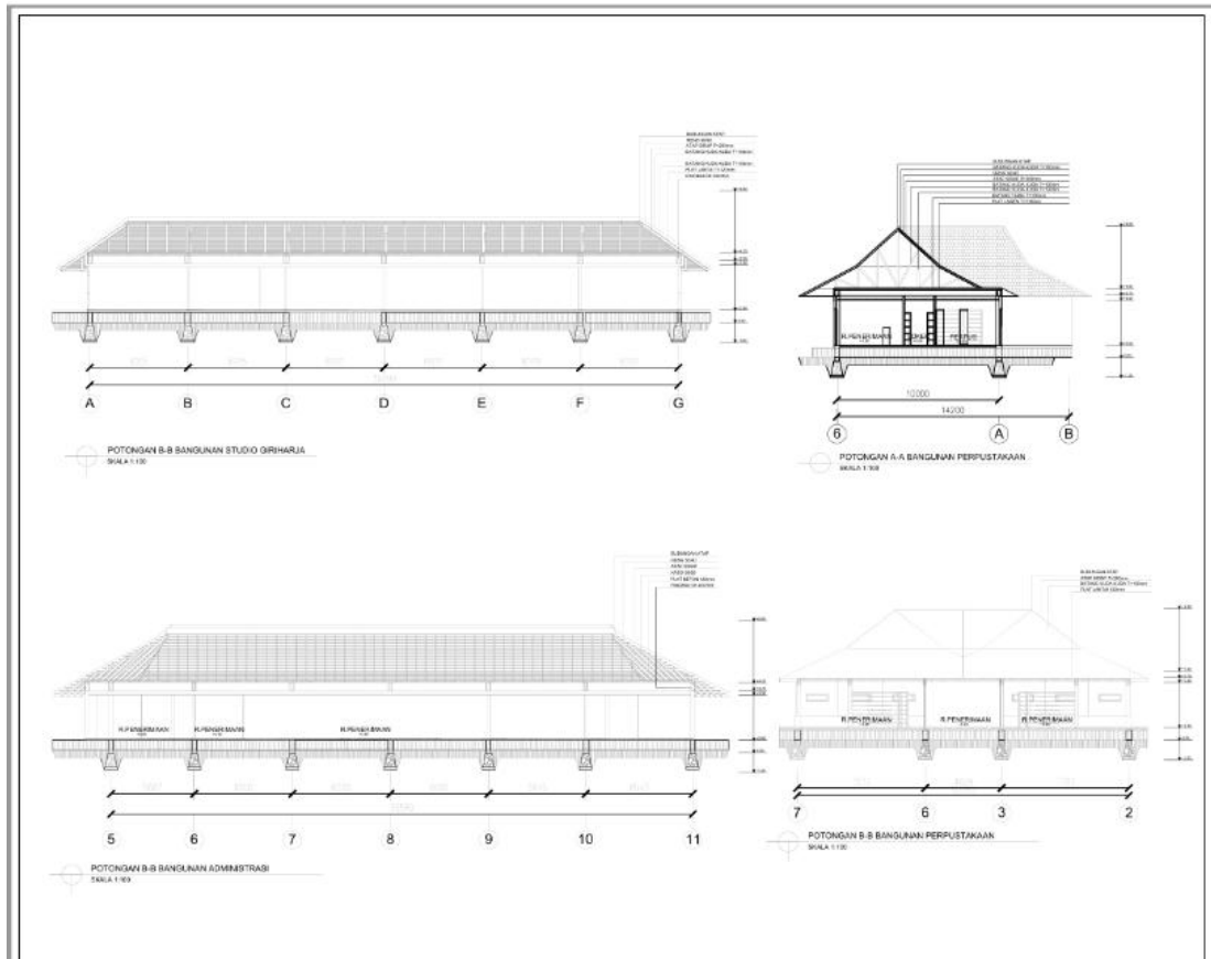
Gambar 6.13 Potongan Sumber : Pribadi
