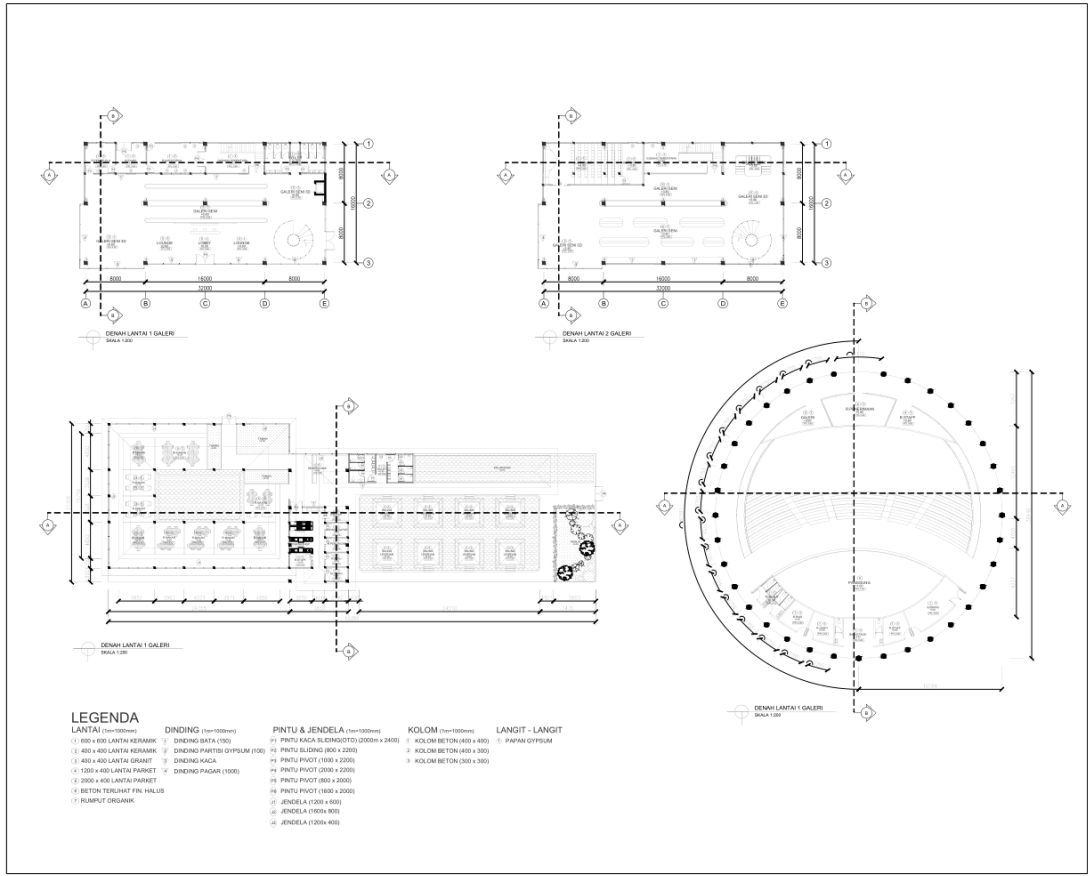
Gambar 6.5 Denah Sumber : Pribadi
