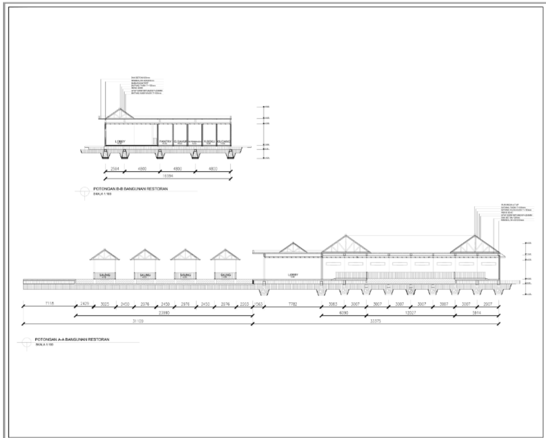
Gambar 6.12 Potongan Sumber : Pribadi
