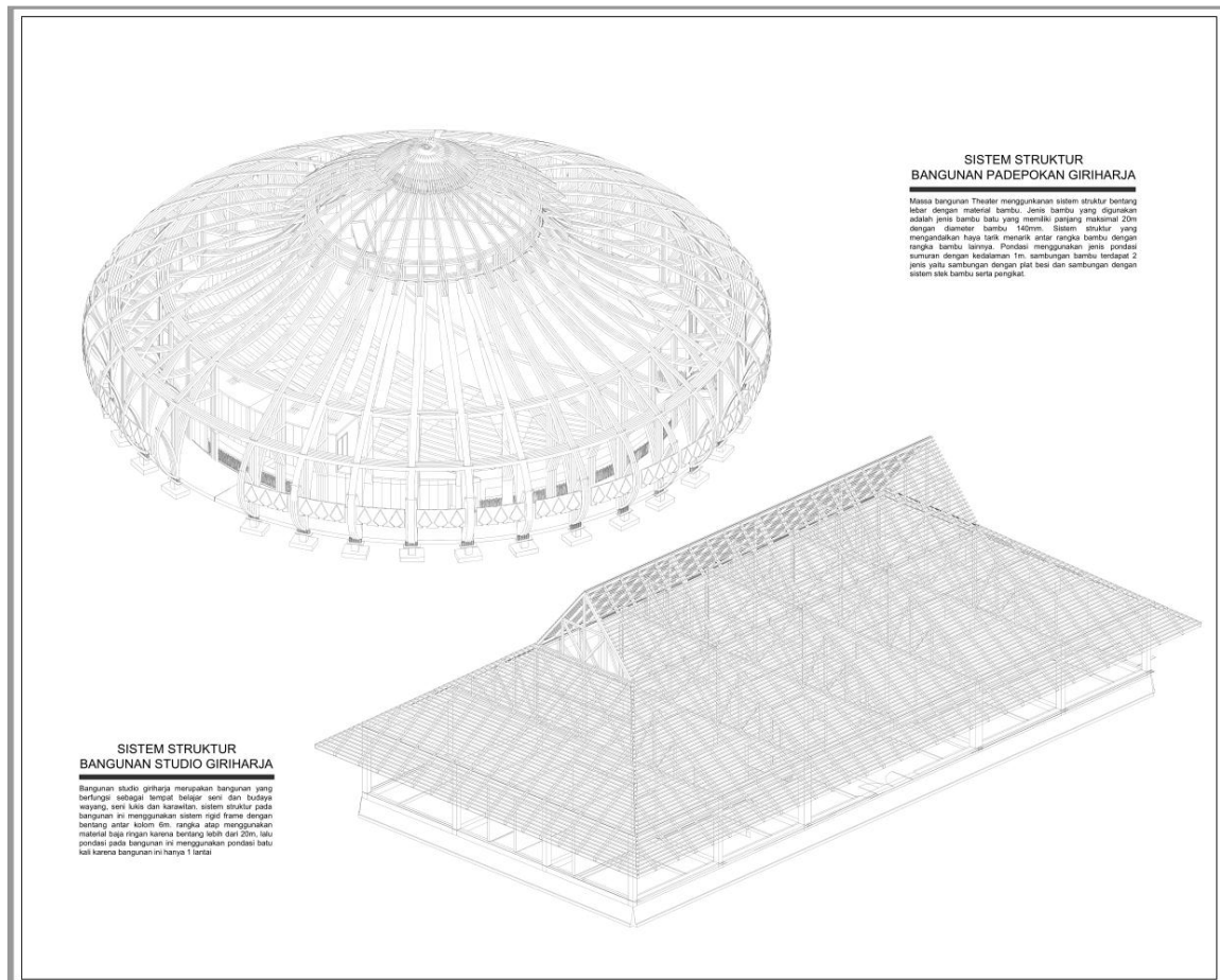
Gambar 6.16 Sistem Struktur Bangunan Sumber : Pribadi
