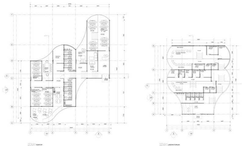
Gambar 6.7 Denah Laboratorium dan kantor
