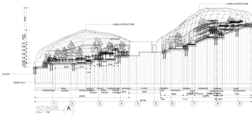
Gambar 6.9 Potongan A Display Teduh
