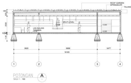
Gambar 6.11 Potongan A dan B Laboratorium
