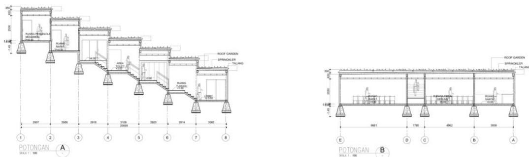
Gambar 6.10 Potongan A dan B Kantor
