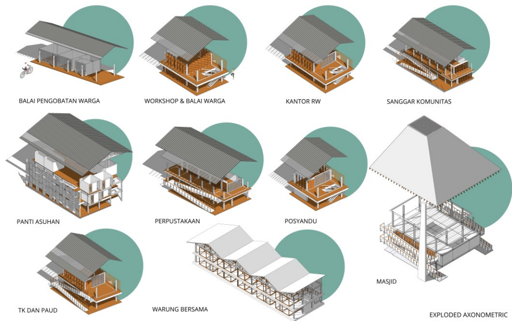
Gambar 6.5. Gambar Perancangan Prototype Bangunan Fasilitas Pendukung
