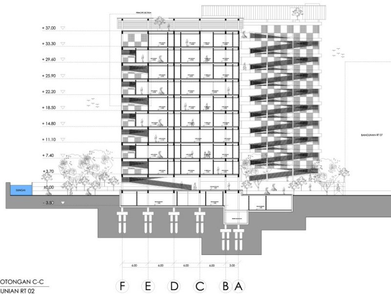
POTONGAN B-B HUNIAN RT 02
