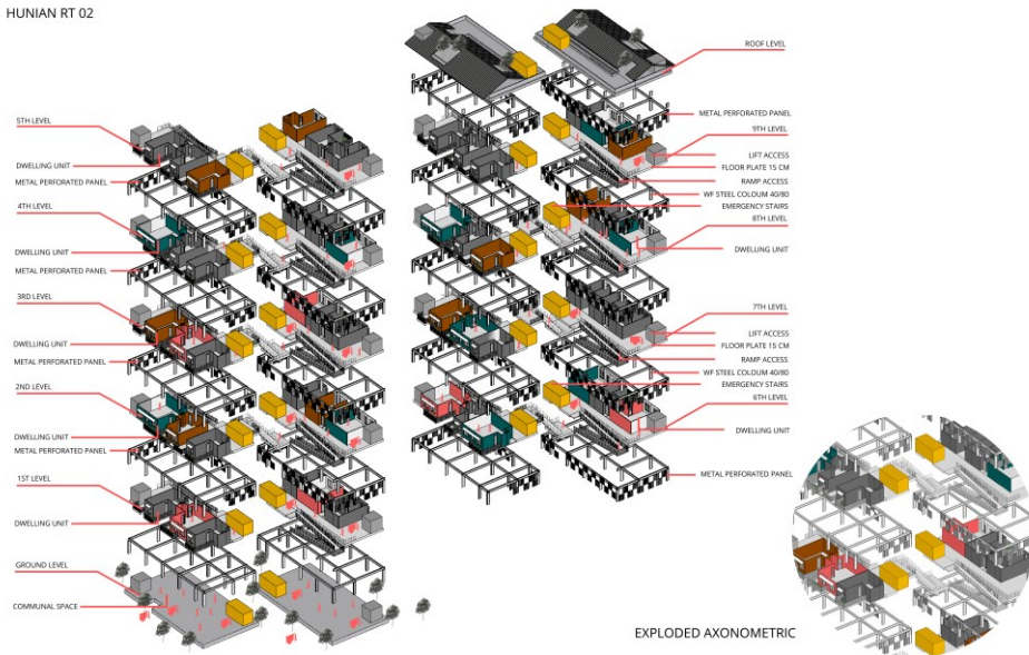
Gambar 6.3. Gambar Perancangan Prototype Bangunan hunian RT 02
