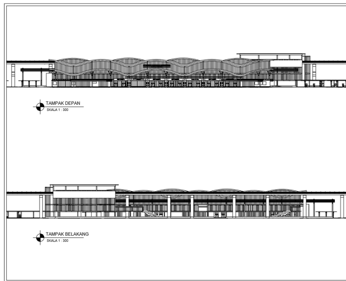
Gambar 6.5 Tampak 1 & 2 (Sumber : Dokumen Pribadi)
