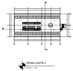
Gambar 6.3 Denah Lantai 3 (Sumber : Dokumen Pribadi)
