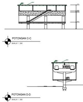
Gambar 6.7 Potongan Stasiun LRT (Sumber : Dokumen Pribadi)
