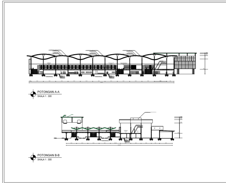
Gambar 6.7 Potongan Stasiun KA (Sumber : Dokumen Pribadi)
