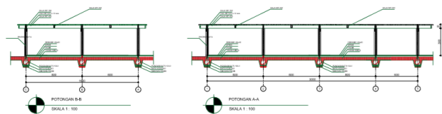
Gambar 6.8 Potongan Bangunan Utilitas (Sumber : Dokumen Pribadi)
