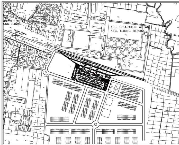
Gambar 6.1 Peta Situasi (Sumber : Dokumen Pribadi)
