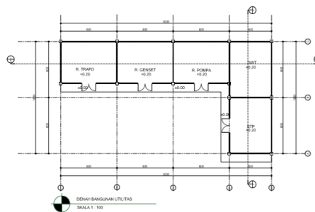
Gambar 6.4 Denah Bangunan Utilitas (Sumber : Dokumen Pribadi)
