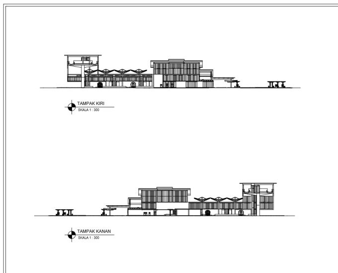
Gambar 6.6 Tampak 3 & 4 (Sumber : Dokumen Pribadi)
