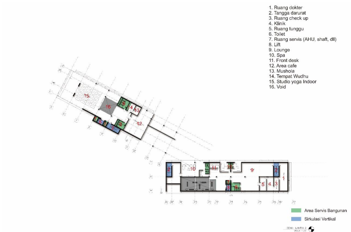
Gambar 0.3 Denah Lantai 2 Sumber ; Dokumen Pribadi
