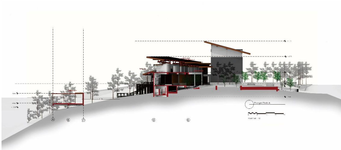
Gambar 0.10 Potongan Site A-A Sumber ; Dokumen Pribadi
