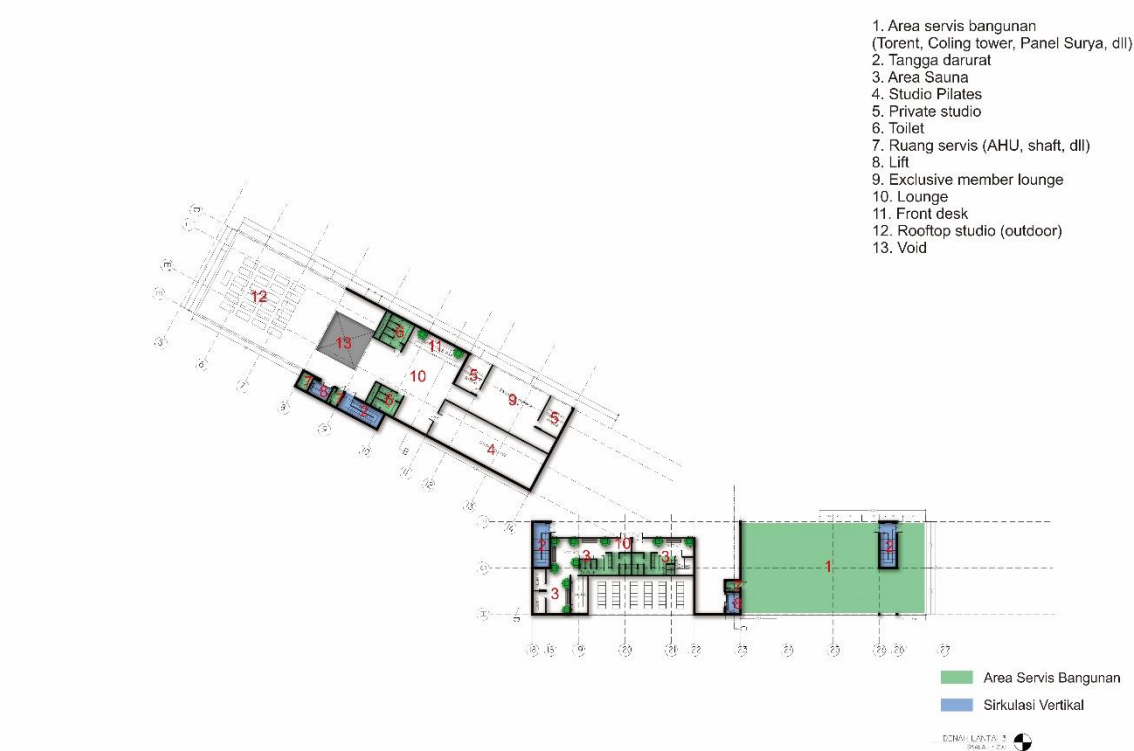
Gambar 0.4 Denah Lantai 3 Sumber ; Dokumen Pribadi
