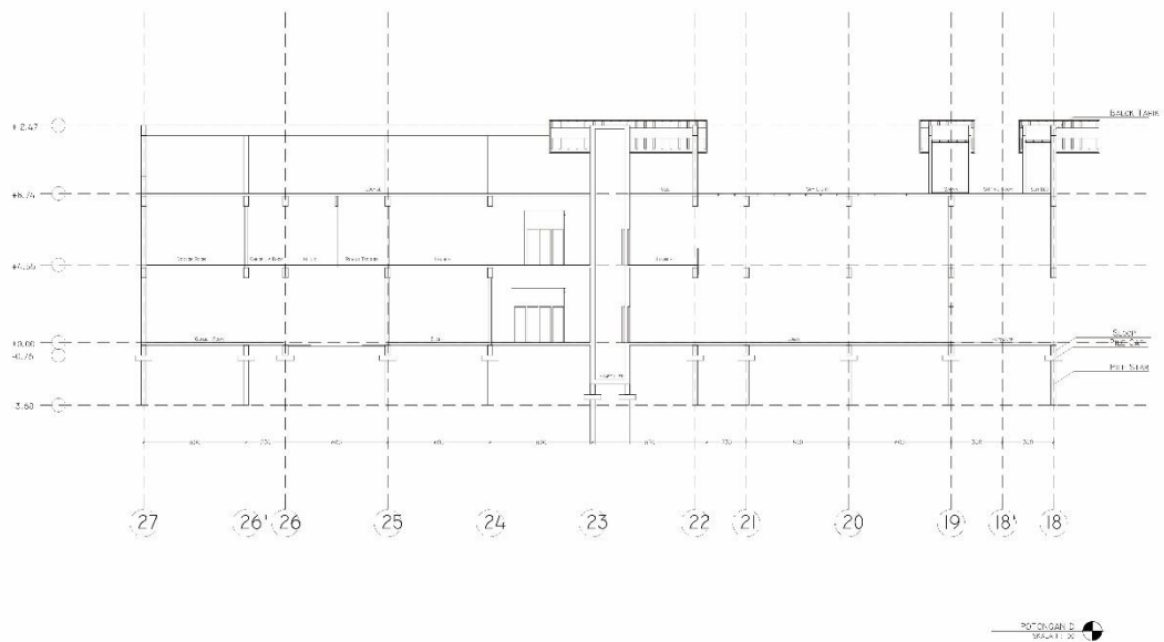
Gambar 0.8 Potongan Prinsip dan Potongan C-C Sumber ; Dokumen Pribadi
