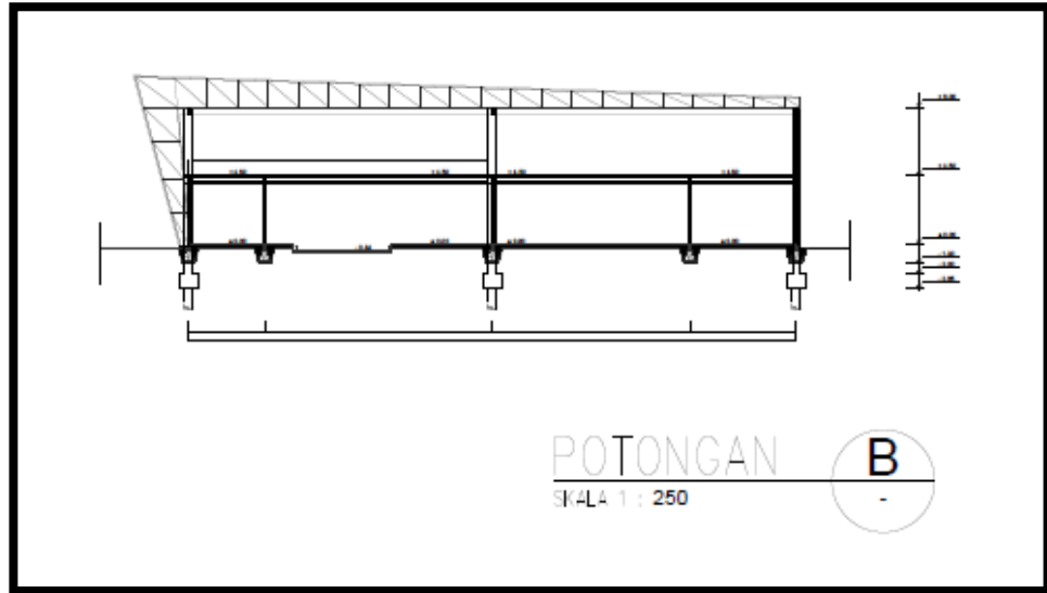
Gambar 6.11. Potongan 2
