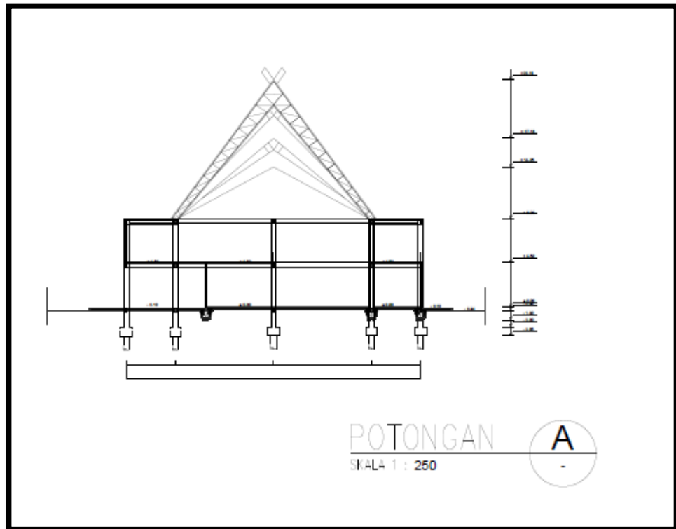
Gambar 6.10. Potongan 1
