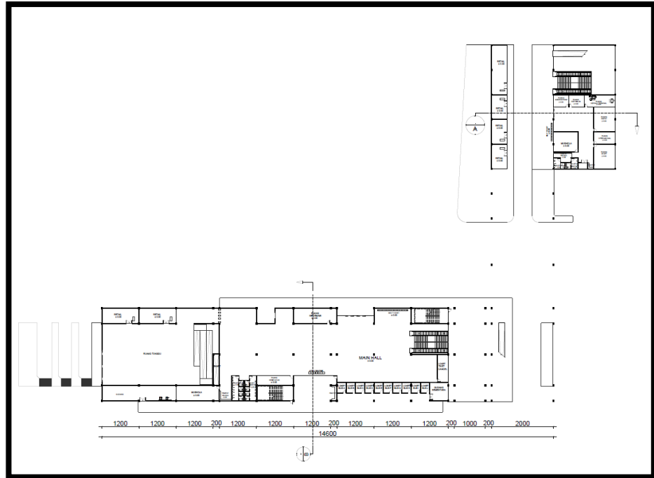
Gambar 6.4. Denah Lantai 1
