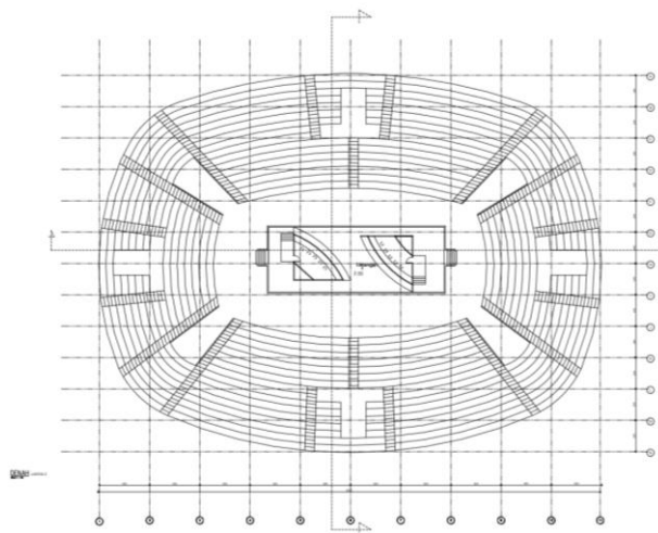
Gambar 6.4 Denah Lantai 2 Lapangan Sumber : Data Pribadi
