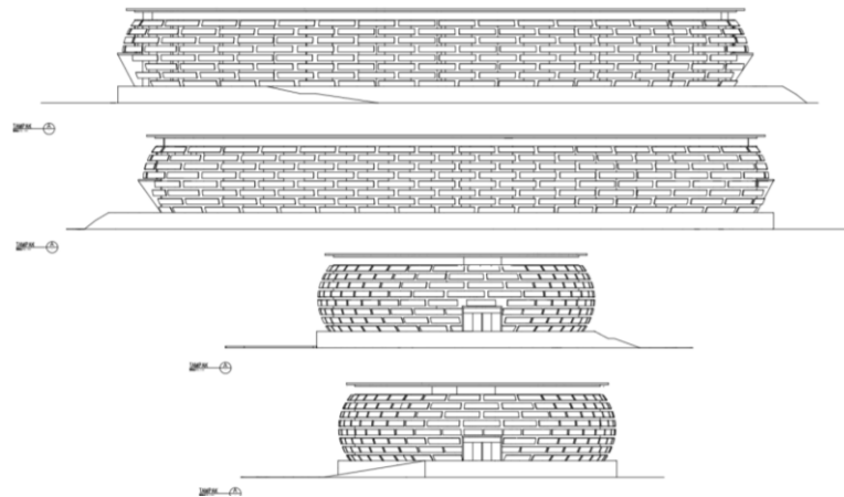
Gambar 6.12 Tampak Retail Sumber : Data Pribadi
