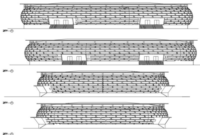
Gambar 6.13 Tampak Lapangan E-sport Sumber : Data Pribadi
