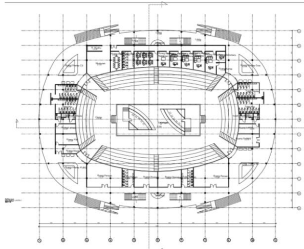
Gambar 6.3 Denah Lantai 1 Lapangan Sumber : Data Pribadi
