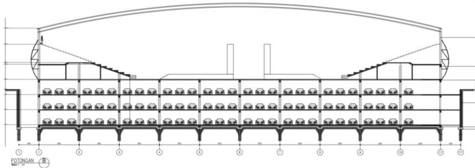
Gambar 6.11 Potongan Lapangan E-Sport Sumber : Data Pribadi
