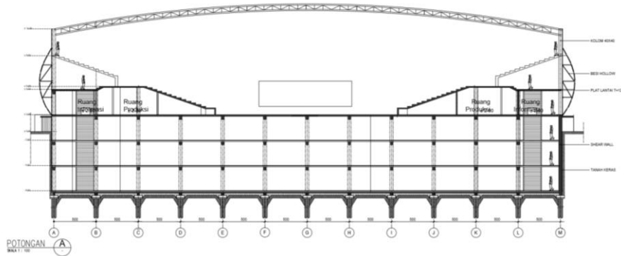
Gambar 6.10 Potongan Retail Sumber : Data Pribadi
