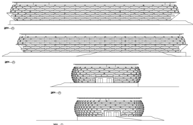
Gambar 6.14 Tampak Foodcourt Sumber : Data Pribadi
