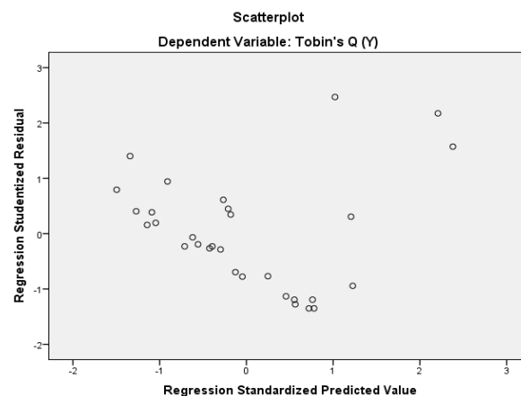
Gambar 2. Uji Heteroskedastisitas
