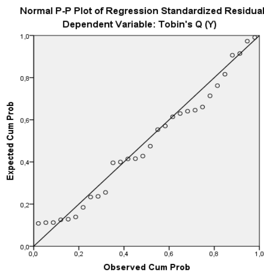
Gambar 1. Uji Normalitas
