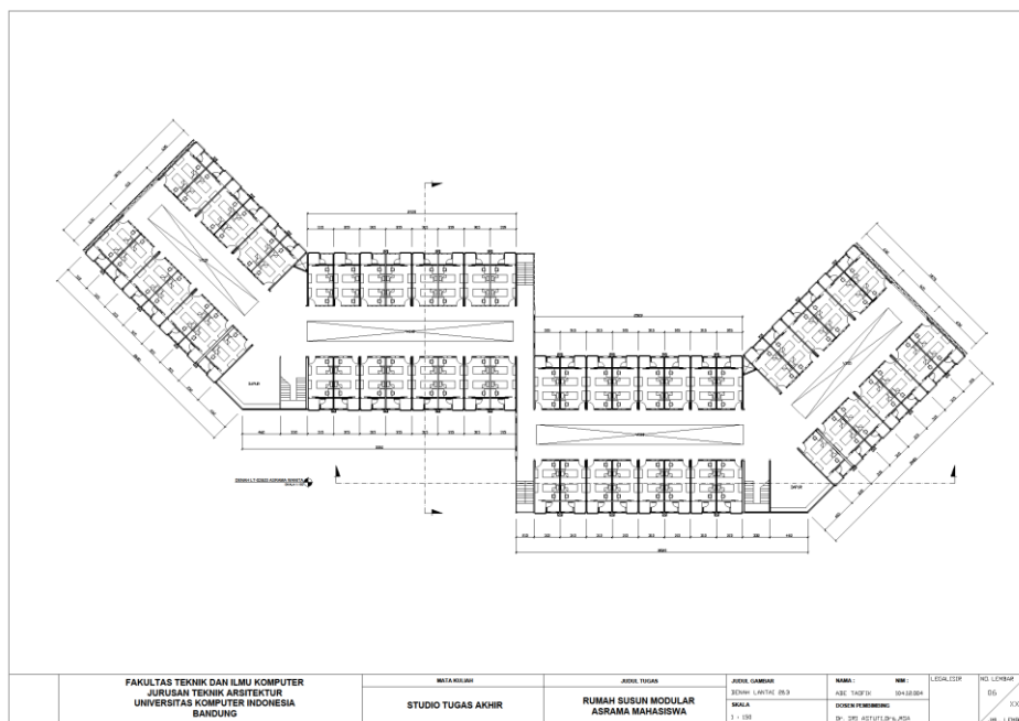
Gambar 6.2.4 Denah Lt-2,3 Asrama Wanita Sumber : Dok. Pribadi
