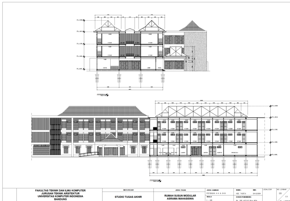
Gambar 6.2.6 Potongan Sumber : Dok. Pribadi
