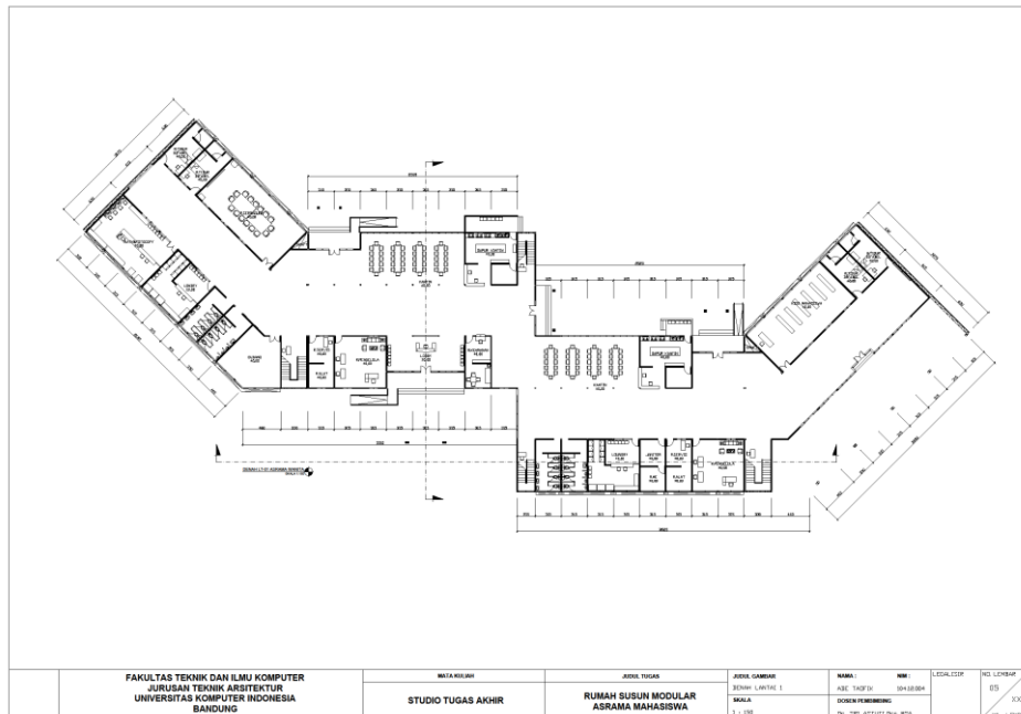
Gambar 6.2.3 Denah Lt-1 Asrama Wanita Sumber : Dok. Pribadi
