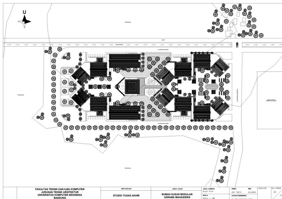
Gambar 6.1.2 Block plan Sumber : Dok. Pribadi
