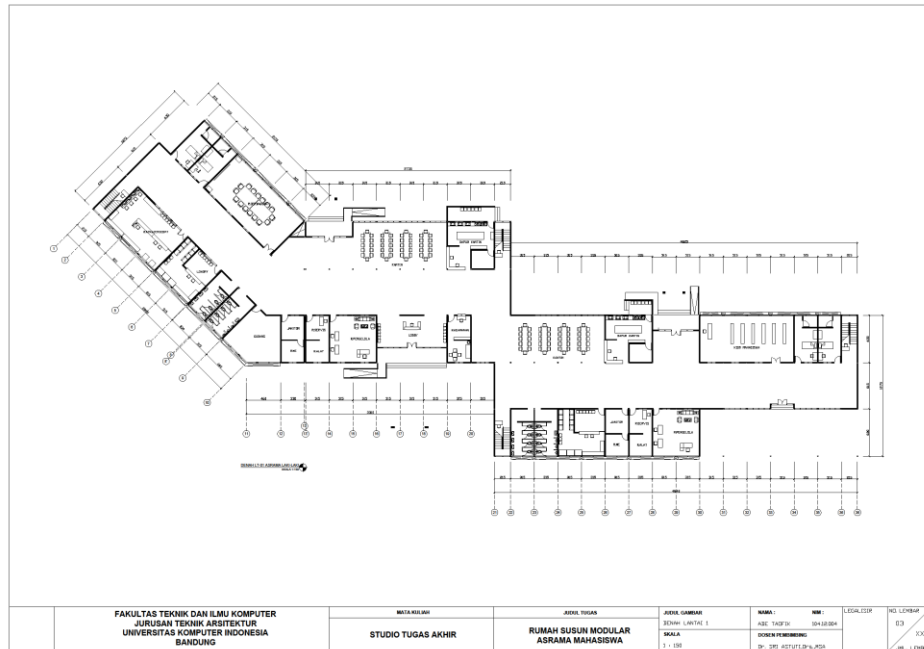
Gambar 6.2.1 Denah Lt-1 Asrama Laki-Laki Sumber : Dok. Pribadi
