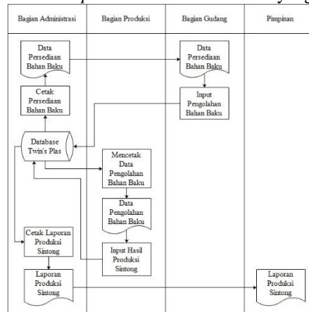
Gambar 2. Flowmap Produksi Sintong yang Diusulkan
