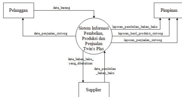
Gambar 4. Diagram Konteks Sistem yang Diusulkan
