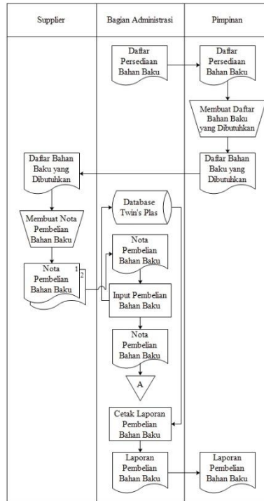
Gambar 1. Flowmap Pembelian Bahan Baku yang Diusulkan
