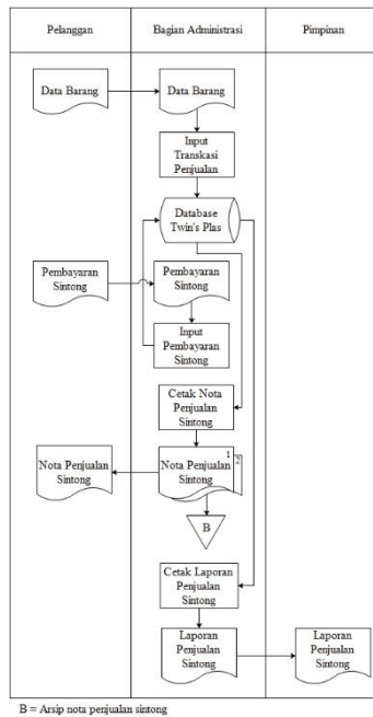
Gambar 3. Flowmap Penjualan Sintong yang Diusulkan
