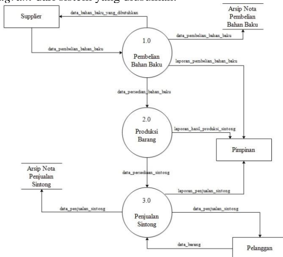
Gambar 5. Data Flow Diagram Level 1 Sistem yang Diusulkan
