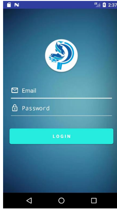
Gambar 4.33 Tampilan LoginActivity
