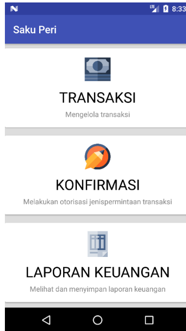
Gambar 4.34 Tampilan MainActivity
