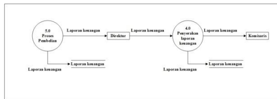
Gambar 5 Data Flow Diagram Level 0 Lanjutan Yang Diusulkan
