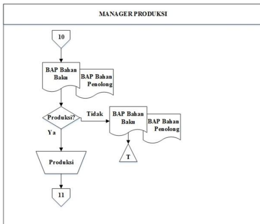
Gambar 13 Flowchat Manager Produksi Yang Diusulkan
