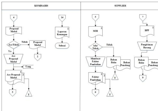
Gambar 12 Flowchat Komisaris & Supplier Yang Diusulkan
