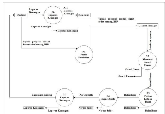
Gambar 11 Data Flow Diagram Level 1 Proses 5 Yang Diusulkan
