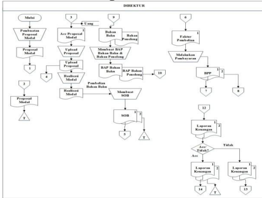
Gambar 11 Flowchat Direktur Yang Diusulkan
