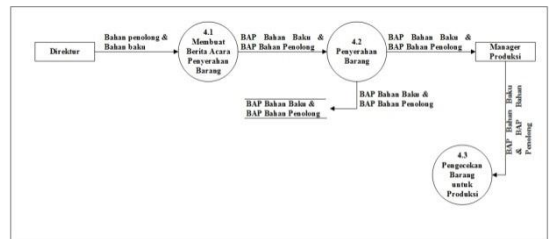
Gambar 10 Data Flow Diagram Level 1 Proses 4 Yang Diusulkan
