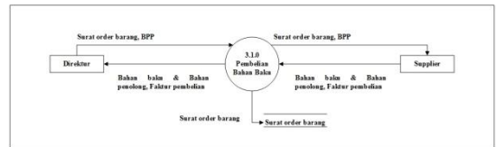
Gambar 8 Data Flow Diagram Level 1 Proses 3 Yang Diusulkan
