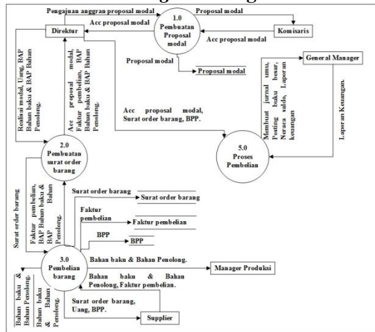
Gambar 4 Data Flow Diagram Level 0 Yang Diusulkan
