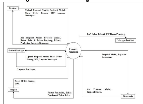
Gambar 3 Diagram Konteks Yang Diusulkan
