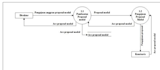
Gambar 6 Data Flow Diagram Level 1 Proses 1 Yang Diusulkan
