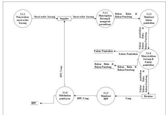
Gambar 9 Data Flow Diagram Level 2 Proses 1 Yang Diusulkan
