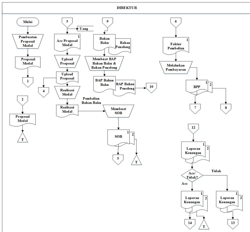
Gambar 4.10 Flowchat Yang Diusulkan 1
