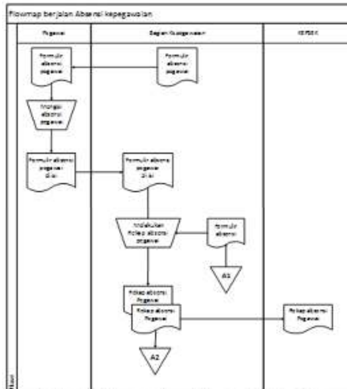
Gambar 2 Flowmap absensi Yang sedang Berjalan
