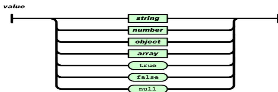
Gambar 2. 7 JSON Value
