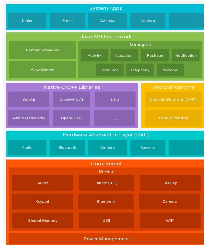
Gambar 2. 3 Arsitektur Android
