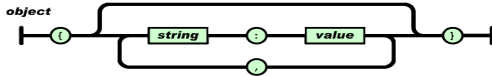
Gambar 2. 5 JSON Object
