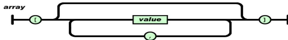
Gambar 2. 6 JSON Array
