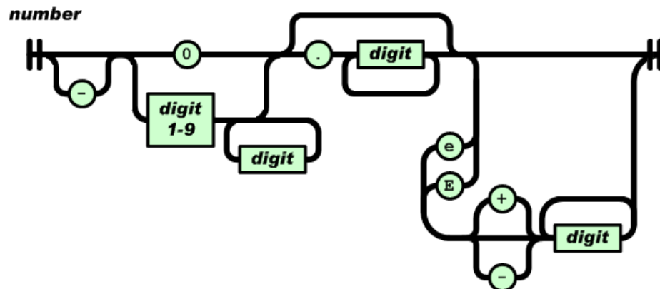
Gambar 2. 9 JSON Angka
