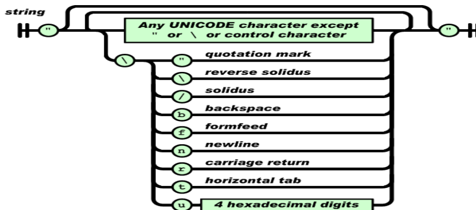
Gambar 2. 8 JSON String
