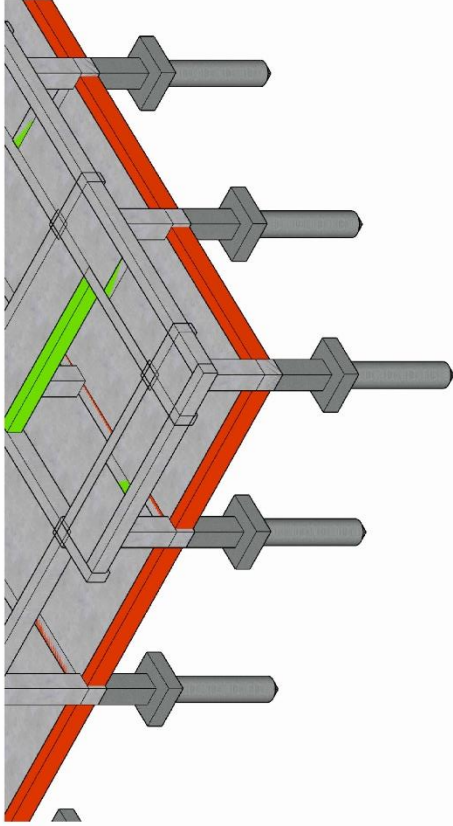
PONDASI TELAPAK
