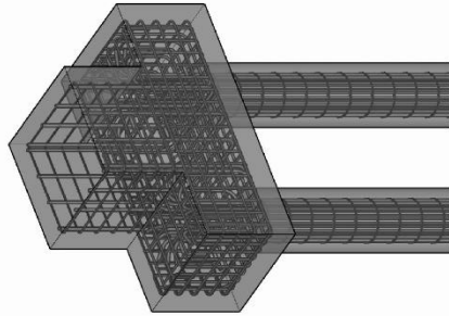
BOREPILE (FONDASI KOLOM STRUKTUR)
