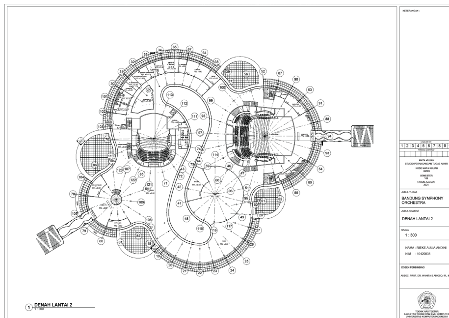
Gambar 34. Denah Lantai 2 Sumber: Dokumentasi Pribadi (2024)
