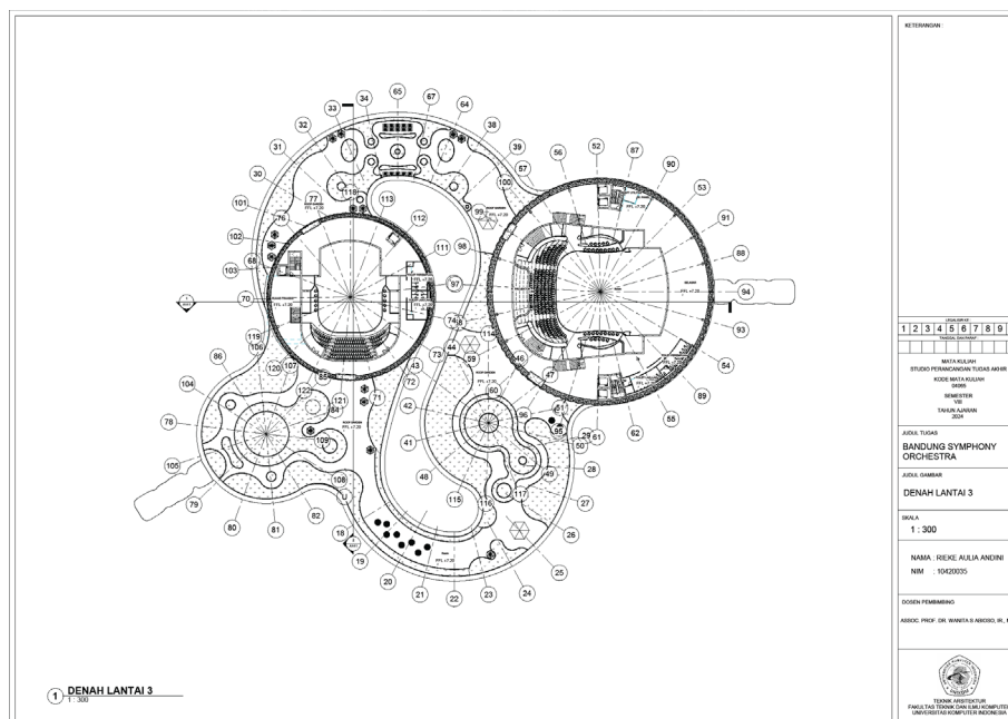
Gambar 35. Denah Lantai 3 Sumber: Dokumentasi Pribadi (2024)
