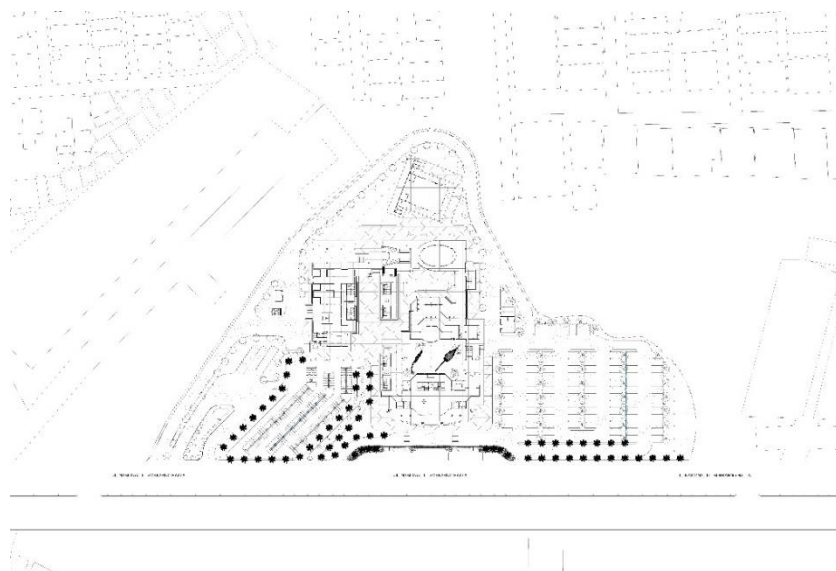
Gambar 46 Gambar Siteplan Sumber: Dokumen Pribadi, 2024
