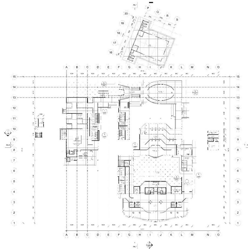
Gambar 47 Denah Lantai 1 Sumber: Dokumen Pribadi, 2024
