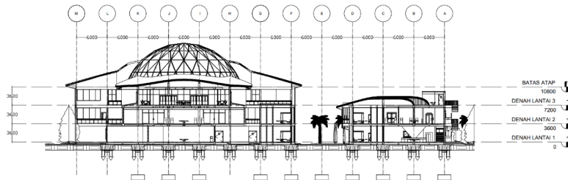
Gambar 51 Potongan Melintang Sumber: Dokumen Pribadi, 2024
