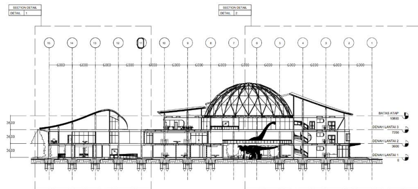
Gambar 50 Potongan Memanjang Sumber: Dokumen Pribadi, 2024
