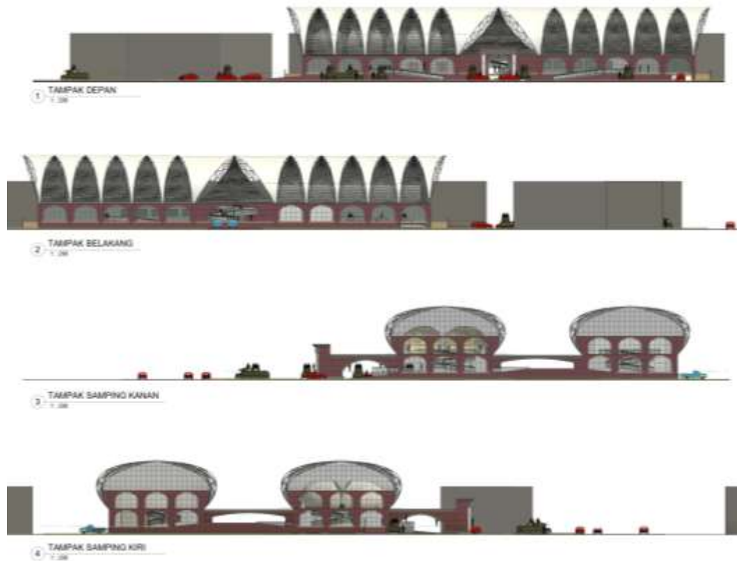
Gambar 6. 4 Tampak Sumber : Data Pribadi
