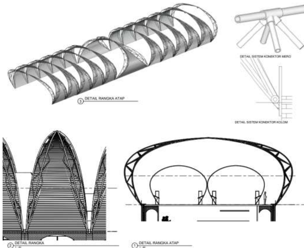
Gambar 6. 7 Detail Arsitektur
