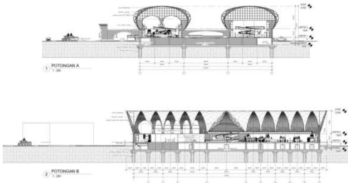
Gambar 6. 5 Potongan Sumber : Data Pribadi
