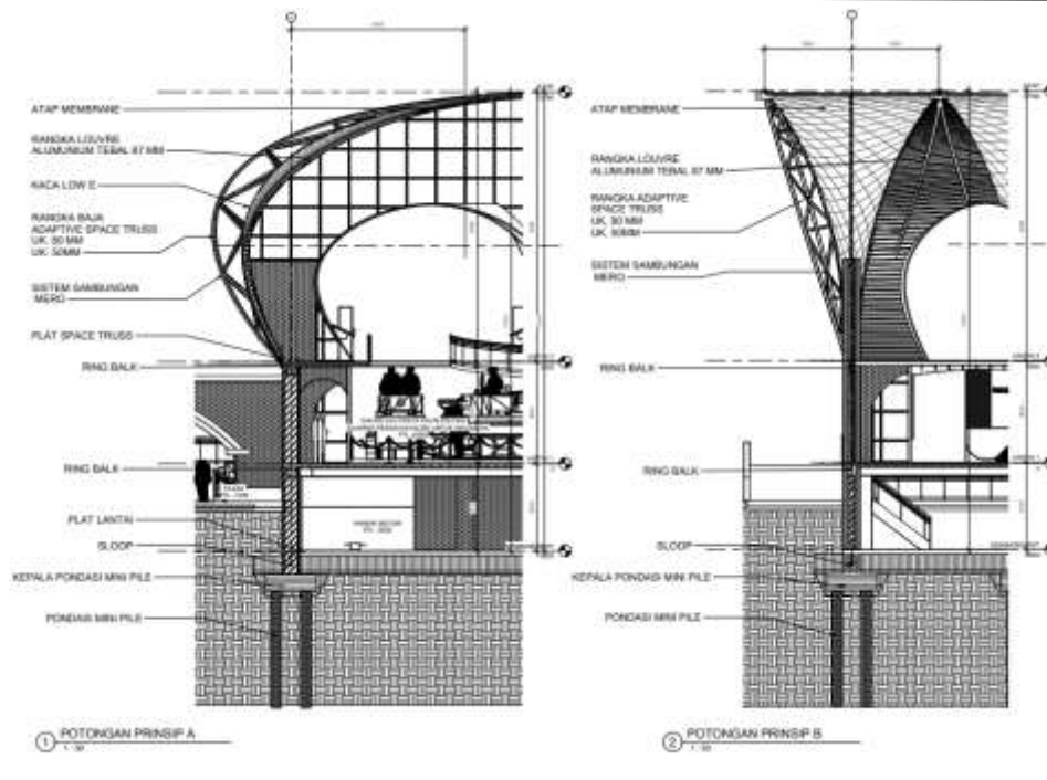
Gambar 6. 6 Potongan Prinsip
