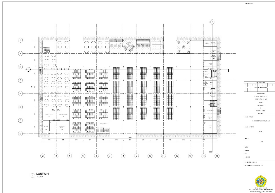
Gambar 36 Denah Lantai 1 (Sumber : Dokumentasi Pribadi)
