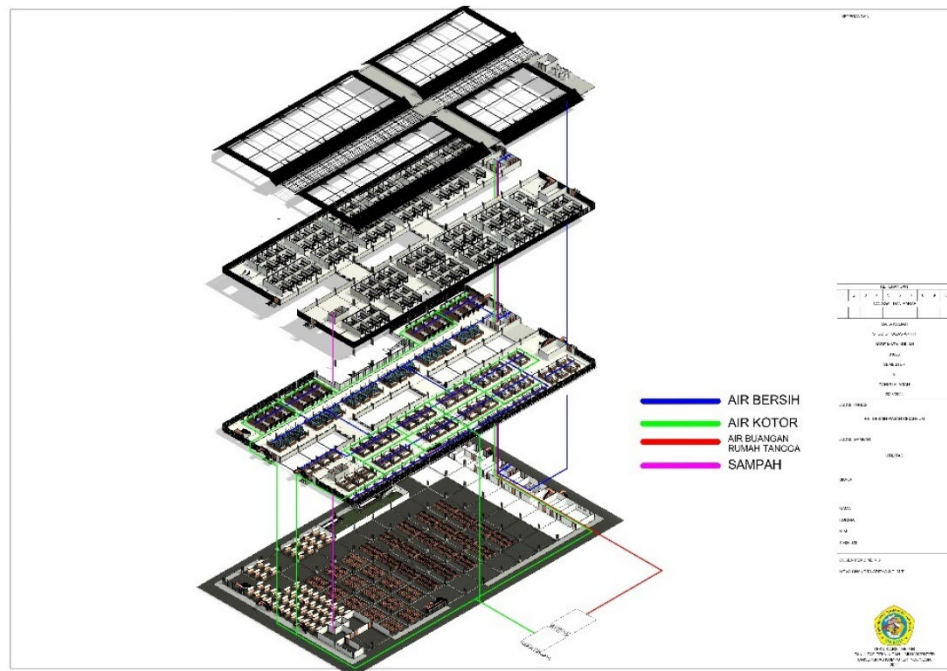
Gambar 56 Sistem Utilitas 1 (Sumber : Dokumentasi Pribadi)
