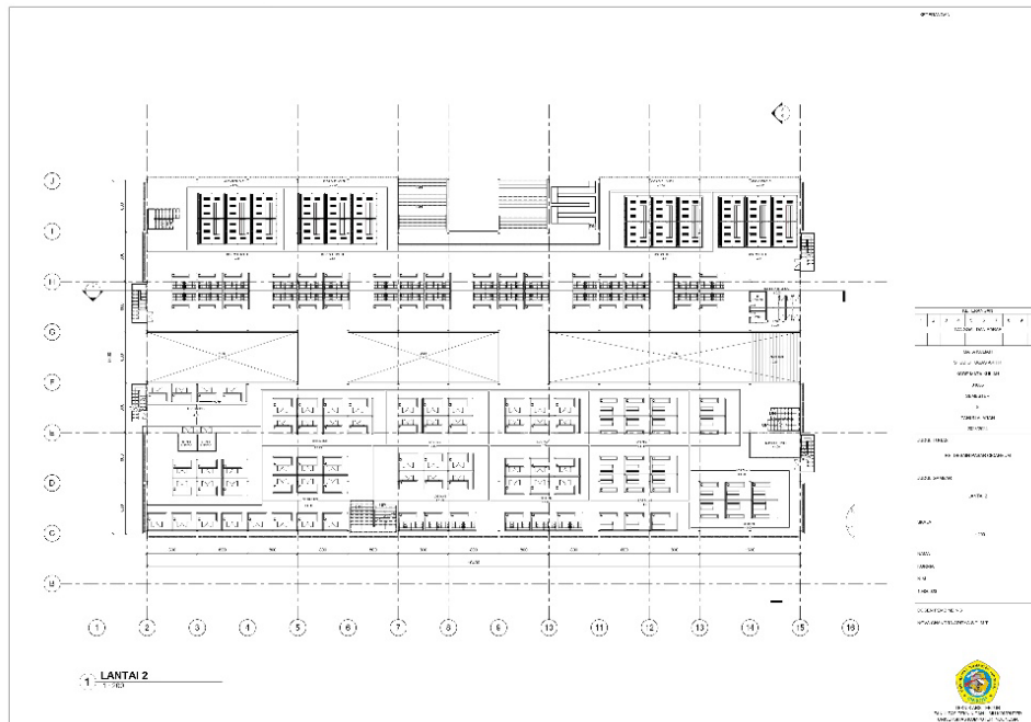
Gambar 37 Denah Lantai 2 (Sumber : Dokumentasi Pribadi)
