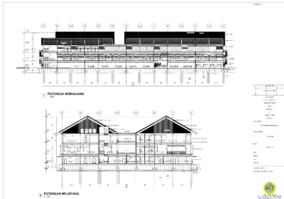
Gambar 40 Potongan A-A dan B-B (Sumber : Dokumentasi Pribadi)
