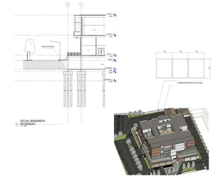
Gambar 6.13 Detail Struktur
