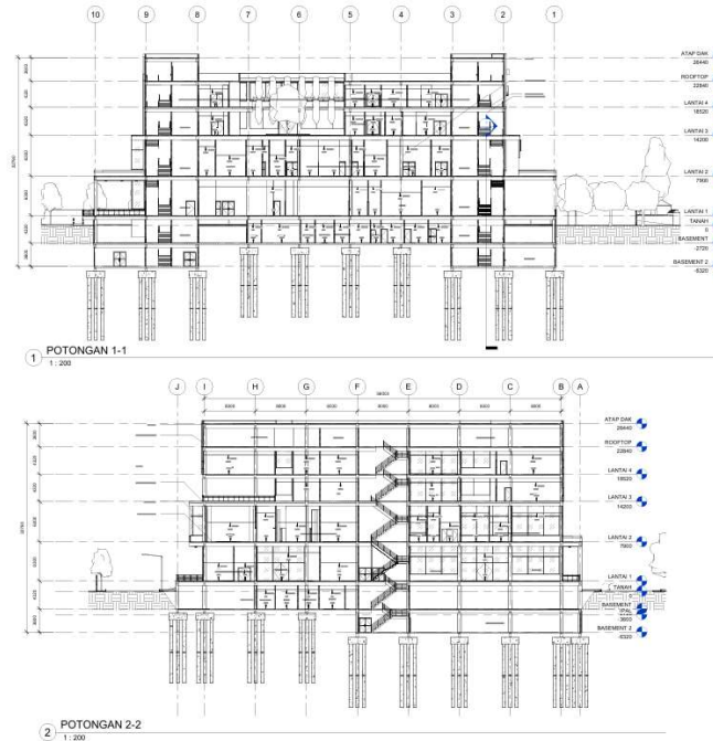
Gambar 6.8 Potongan
