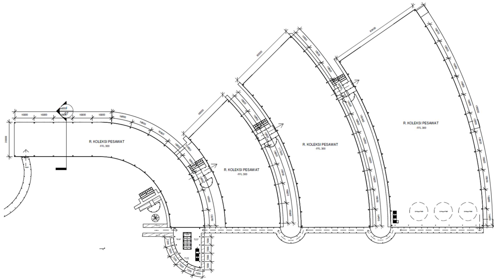
Gambar 6. 4 Denah Gd. Koleksi Pesawat & F&B
