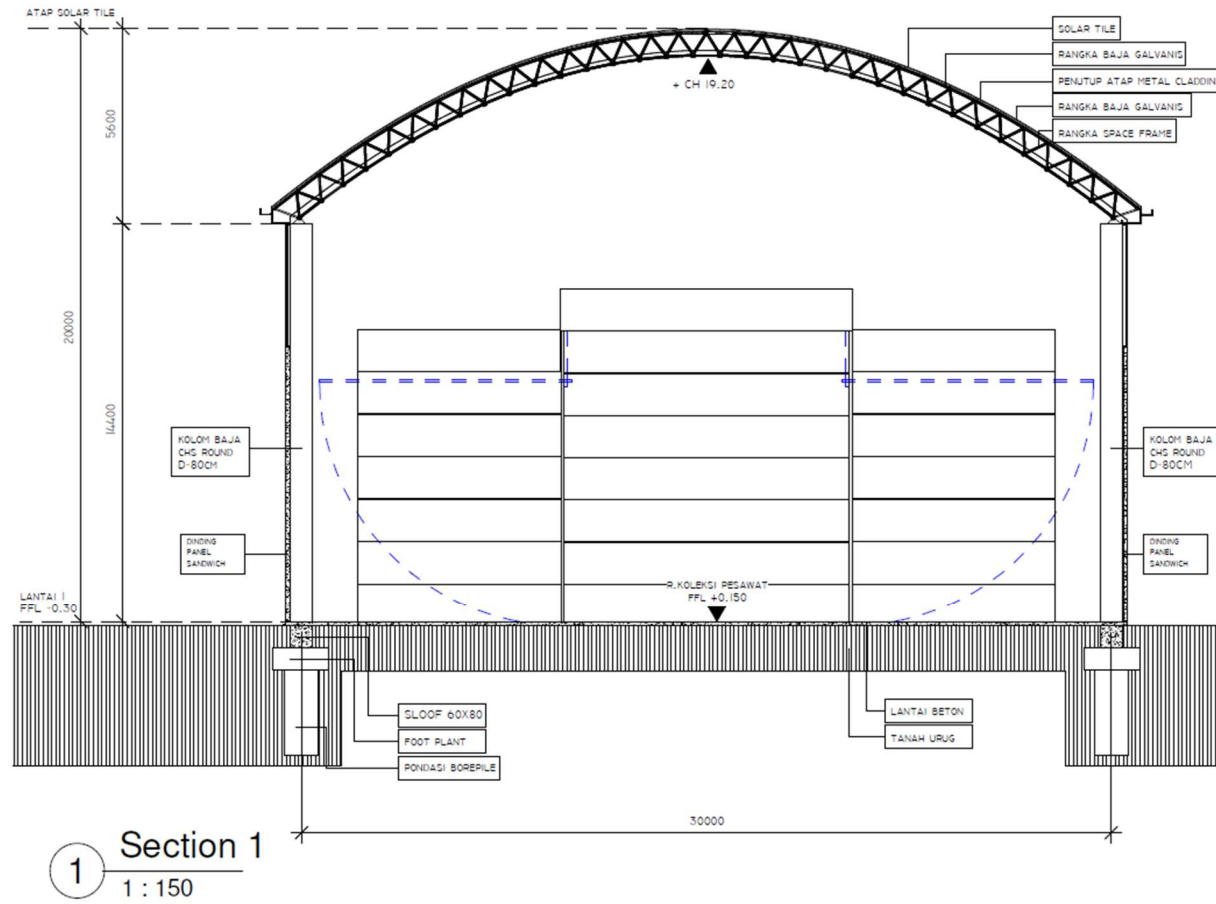
Gambar 6. 10 Potongan A
