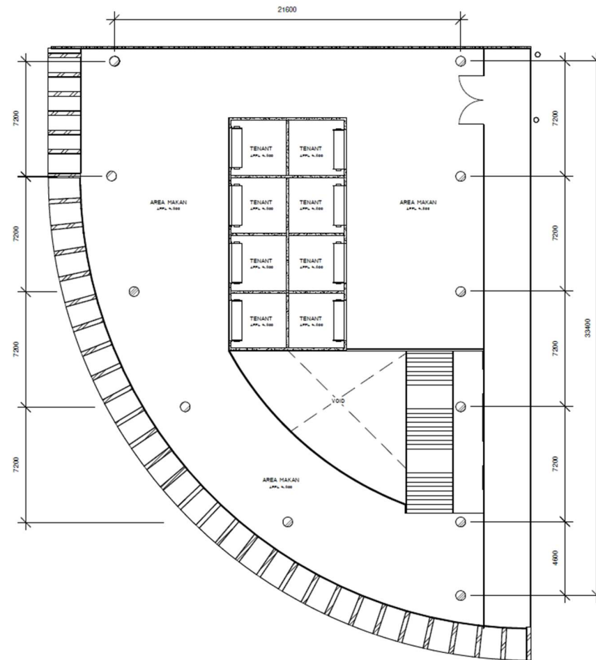
Gambar 6. 8 Denah Lt.2 Gd. F& B
