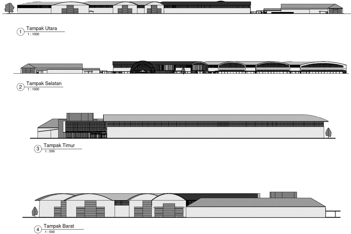
Gambar 6. 9 Tampak
