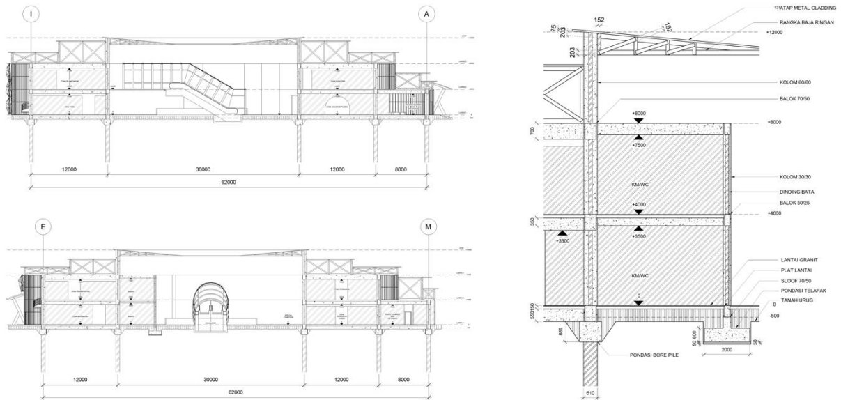
Gambar 6.11 Potongan Bangunan A Museum Sains dan Inovasi Teknologi
