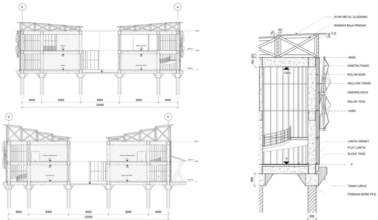
Gambar 6.12 Potongan Bangunan B Museum Sains dan Inovasi Teknologi
