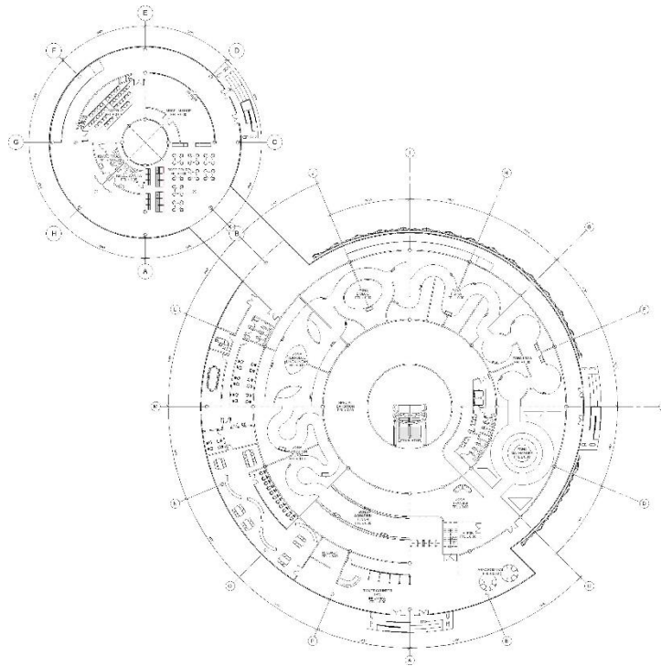
Gambar 6.3 Denah Lt.1 Bangunan Museum Sains dan Inovasi Teknologi
