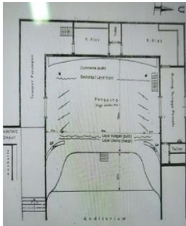
Gambar 2. 6 Denah rumentang siang (Sumber: Dokumen pribadi)
