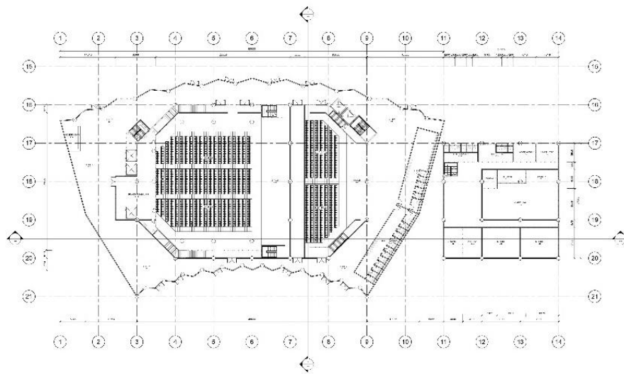
Gambar 6. 5 Denah lantai 2 (Sumber: Dokumen pribadi)
