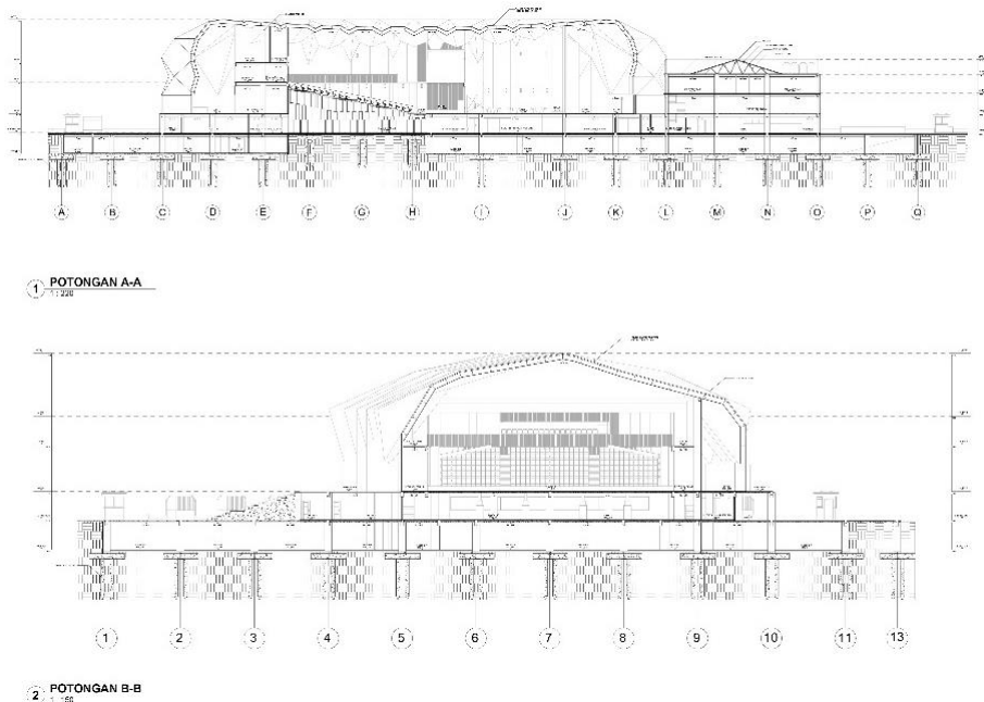
Gambar 6. 8 Potongan (Sumber: Dokumen pribadi)
