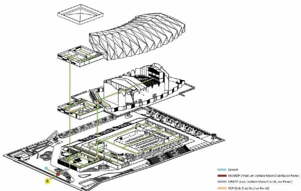
Gambar 6. 12 Utilitas listrik (Sumber: Dokumen pribadi)
