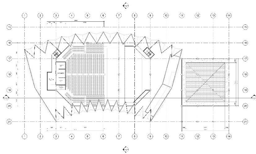
Gambar 6. 7 Denah lantai 4 (Sumber: Dokumen pribadi)
