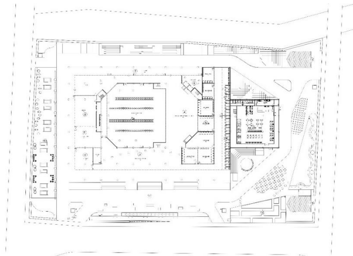
Gambar 6. 2 Siteplan (Sumber: Dokumen pribadi)
