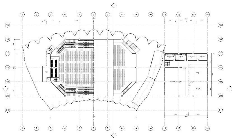
Gambar 6. 6 Denah lantai 3 (Sumber: Dokumen pribadi)
