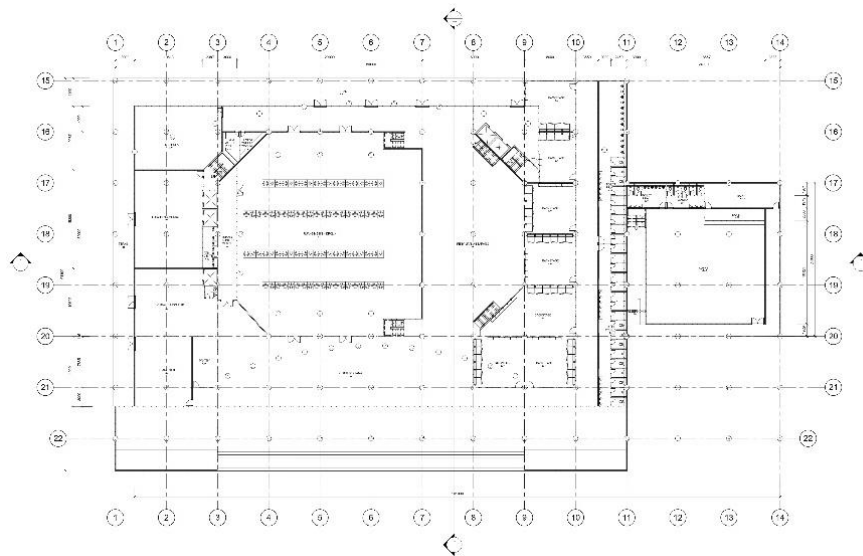
Gambar 6. 4 Denah lantai 1 (Sumber: Dokumen pribadi)
