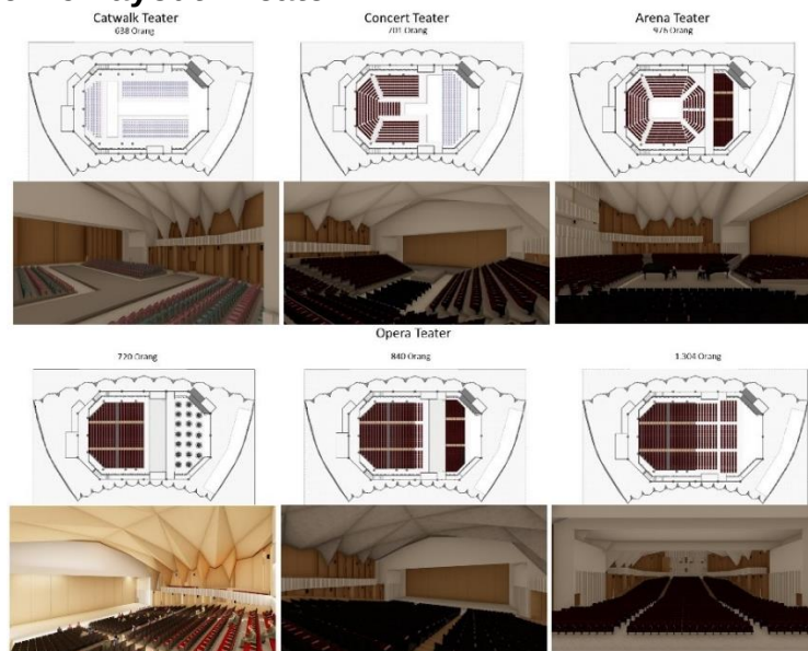
Gambar 6. 15 Layout teater (Sumber: Dokumen pribadi)
