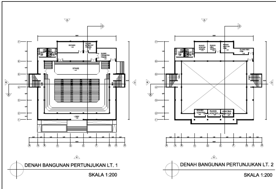
Gambar 6.3 Denah Bangunan Pertunjukan
