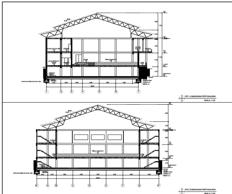
Gambar 6.5 Potongan Bangunan Pertunjukan
