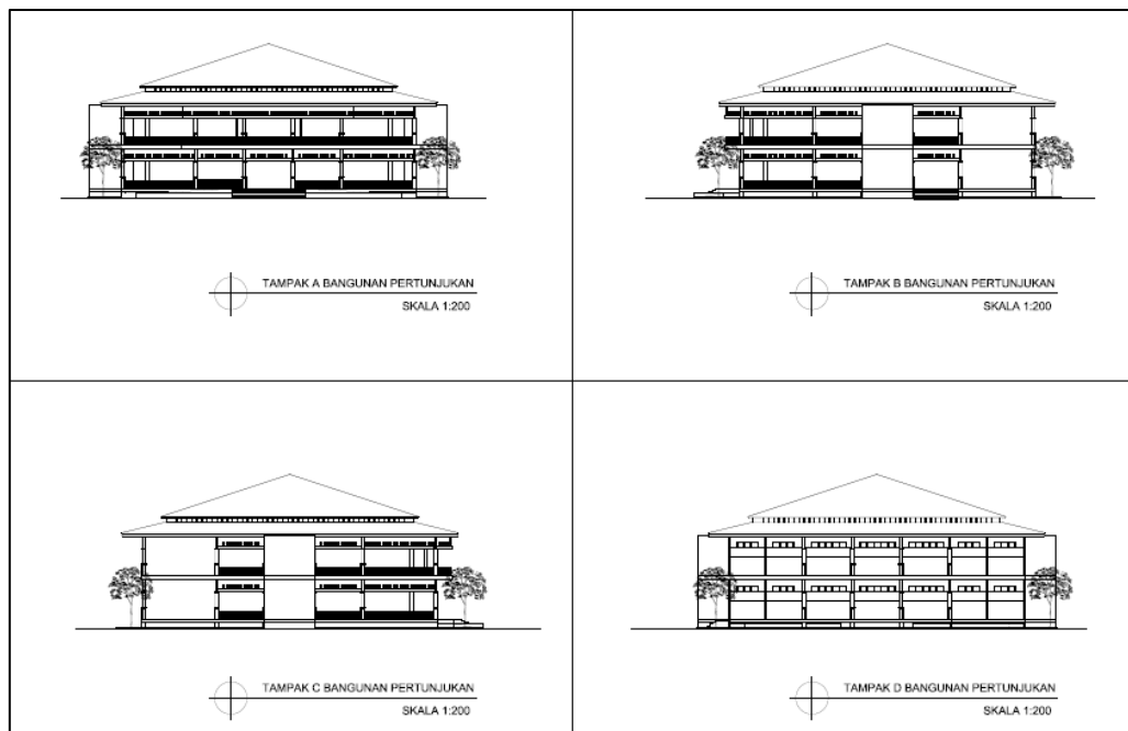
Gambar 6.4 Tampak Bangunan Pertunjukan
