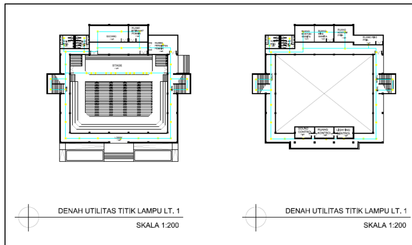
Gambar 6.7 Rencana Instalasi Elektrikal
