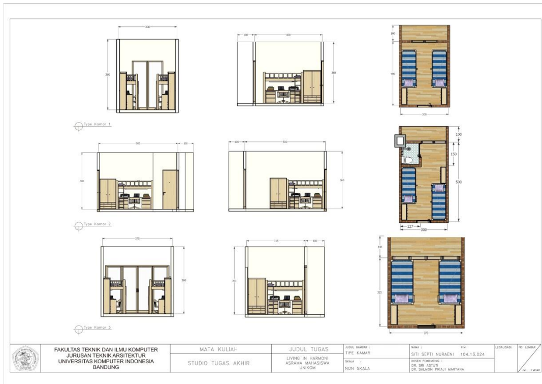
Gambar 6.17 Tipe Kamar
