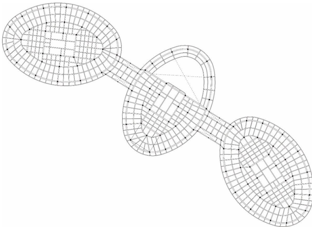
Gambar 6.8. Sistem Pembalokan dan Struktur Bangunan Toyota Automobile Museum Center
