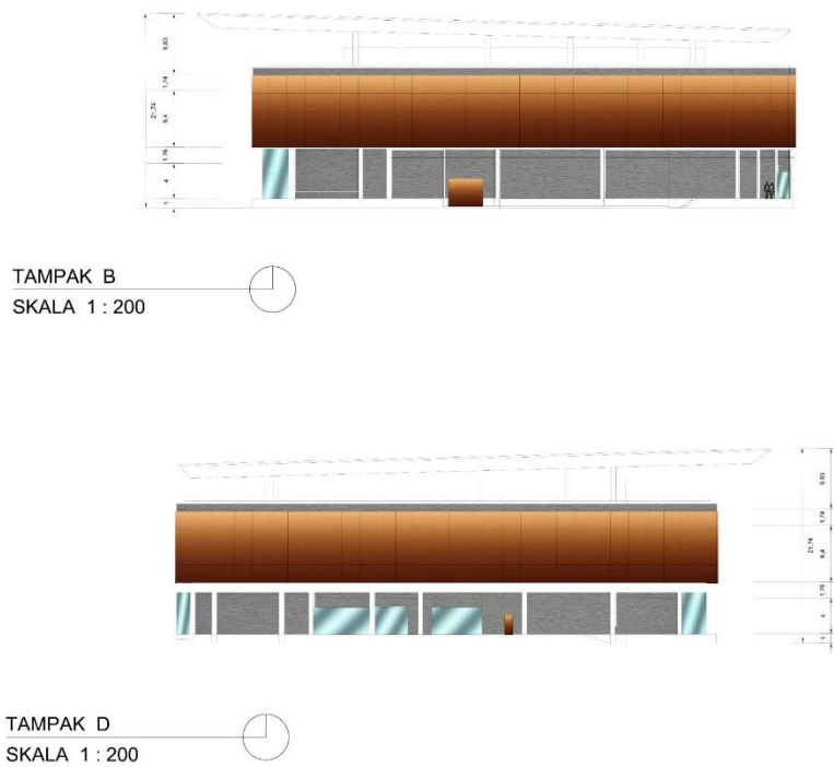
Gambar 6.6. Tampak Samping kanan Dan Samping Kiri Bangunan Toyota Automobile Museum Center
