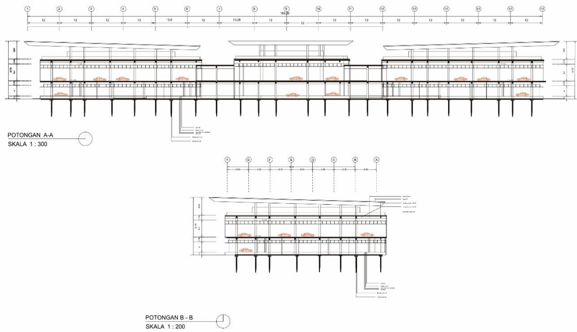
Gambar 6.7. Potongan Bangunan Toyota Automobile Museum Center
